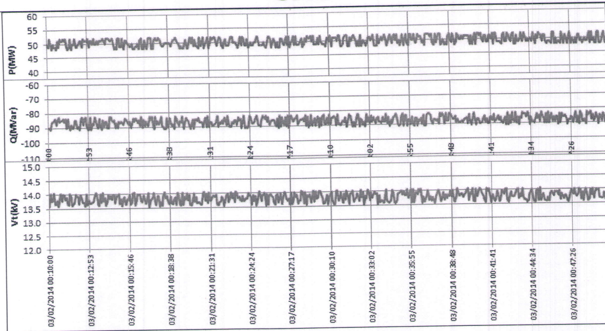
Figura 6-14: Registro Región Subexcitación – Mínimo Técnico
