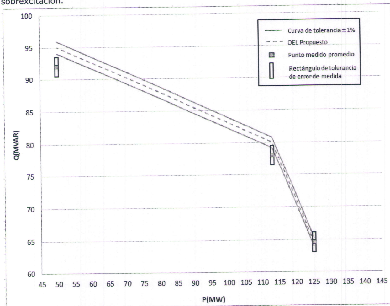
Figura 6-2 Detalle de actuación OEL
