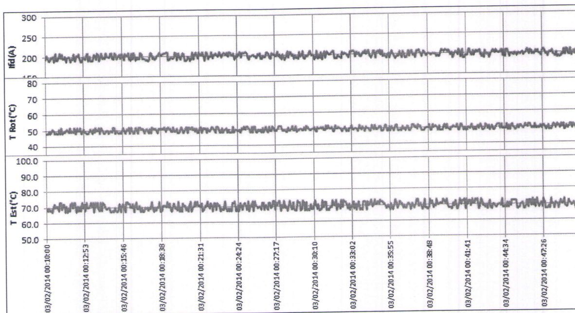
Figura 6-13: Registro Región Subexcitación – Carga Media
