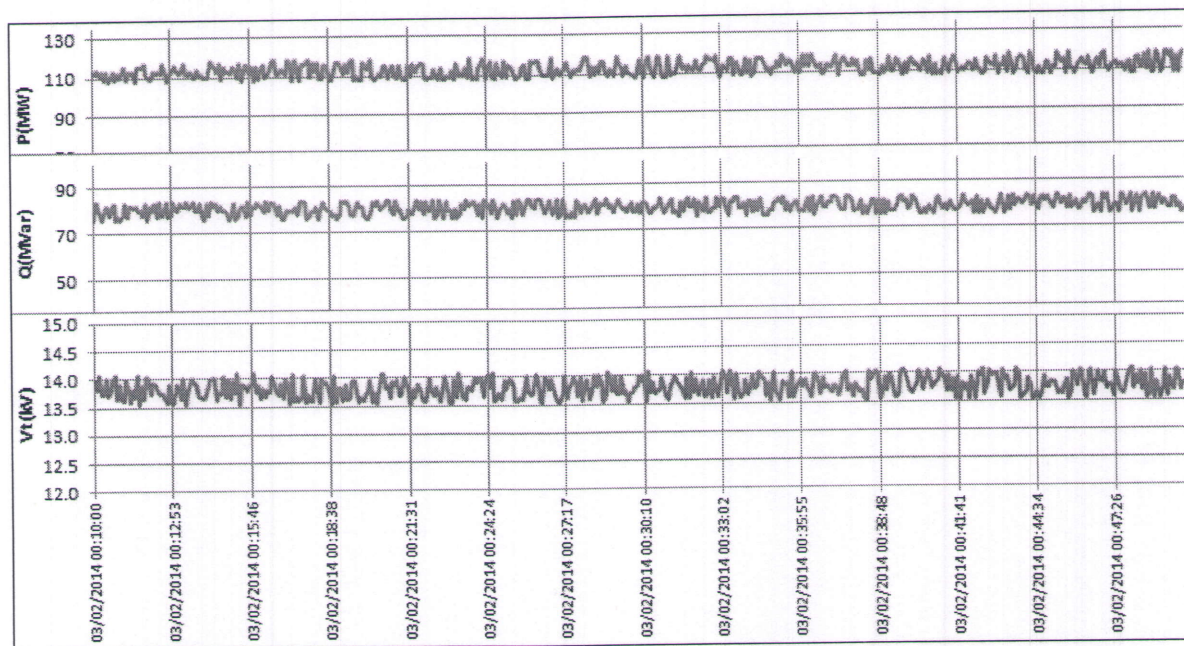
Figura 6-6: Registro Región Sobreexcitación – Carga Media
