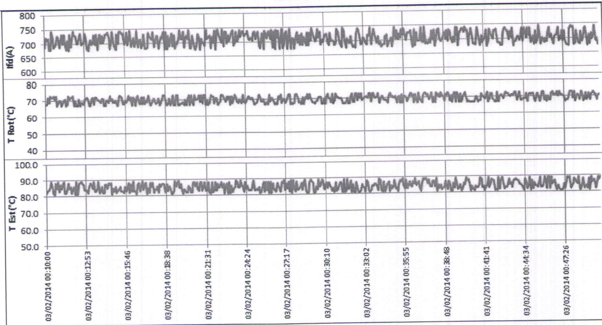
Figura 6-7: Registro Región Sobreexcitación – Carga Media
