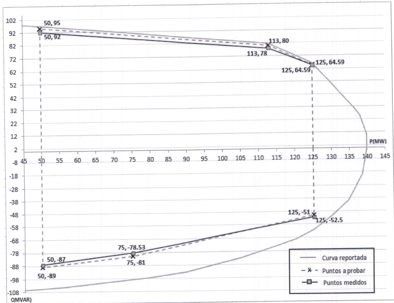
Figura 6-1 Curva de capacidad verificada
