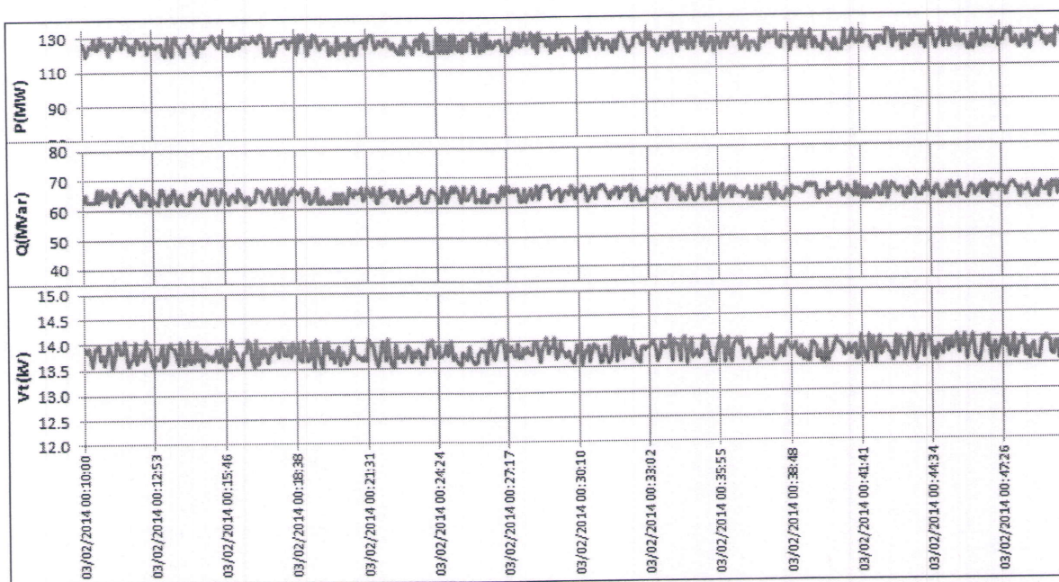
Figura 6-4: Registro Región Sobreexcitación –Carga Alta
