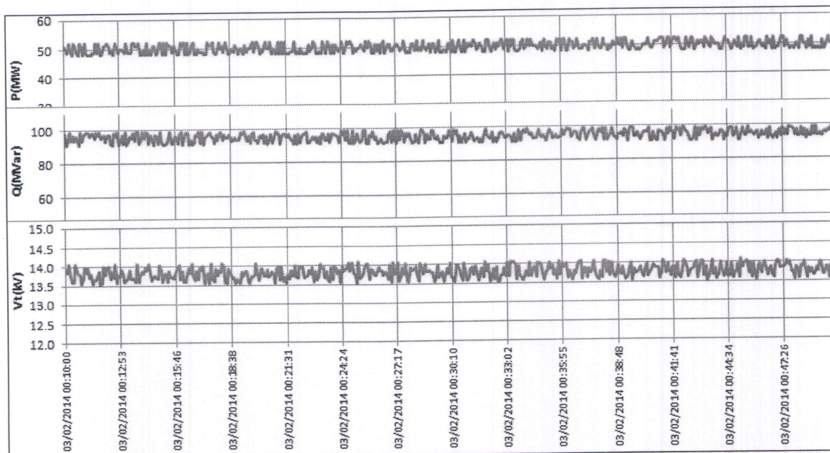
Figura 6-8: Registro Región Sobreexcitación – Mínimo Técnico
