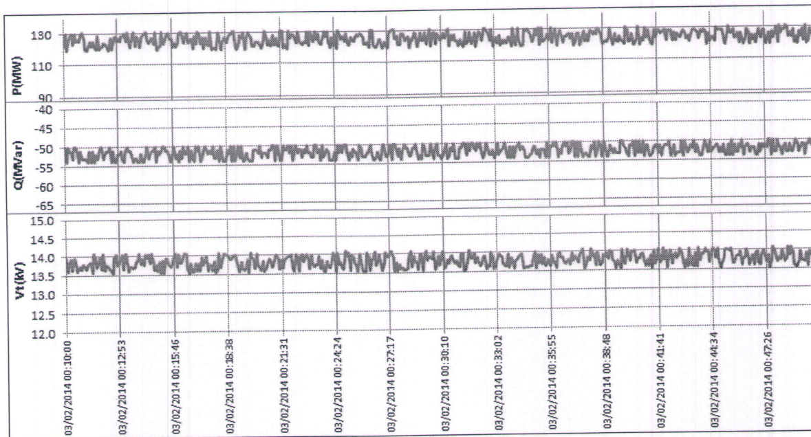
Figura 6-10: Registro Región Subexcitación – Potencia Nominal
