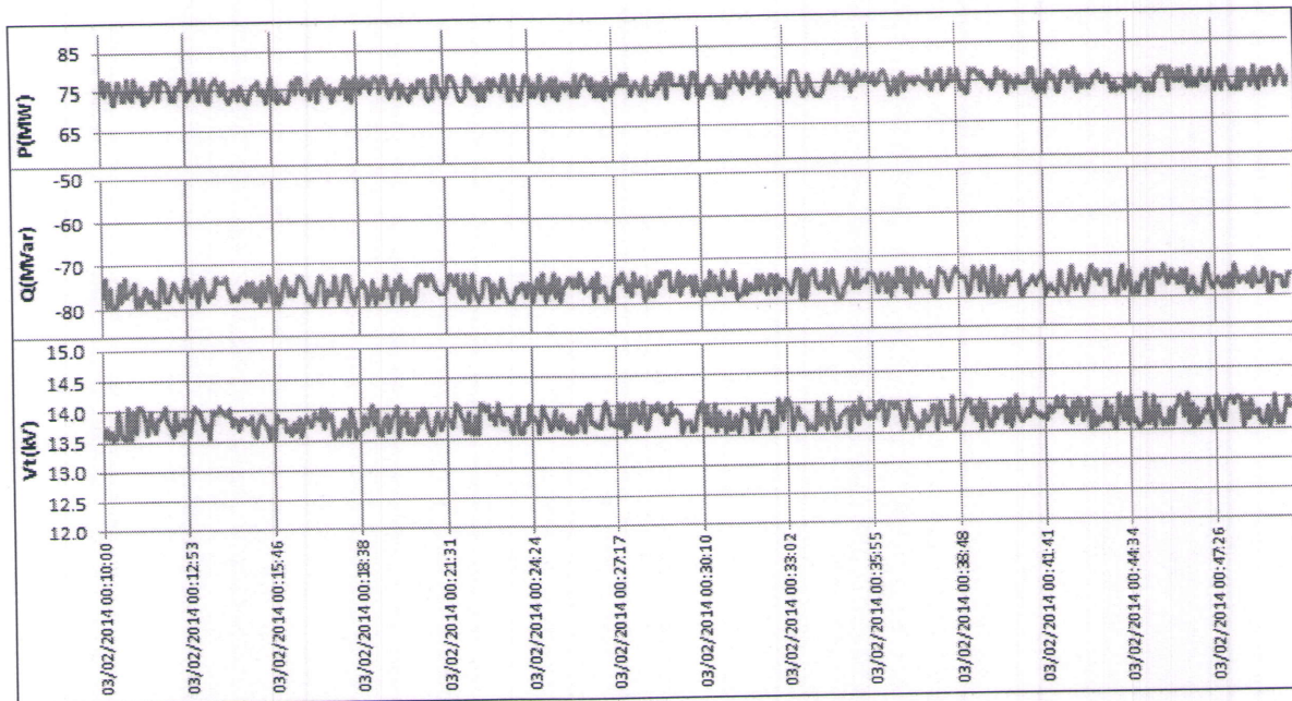
Figura 6-12: Registro Región Subexcitación – Carga Media
