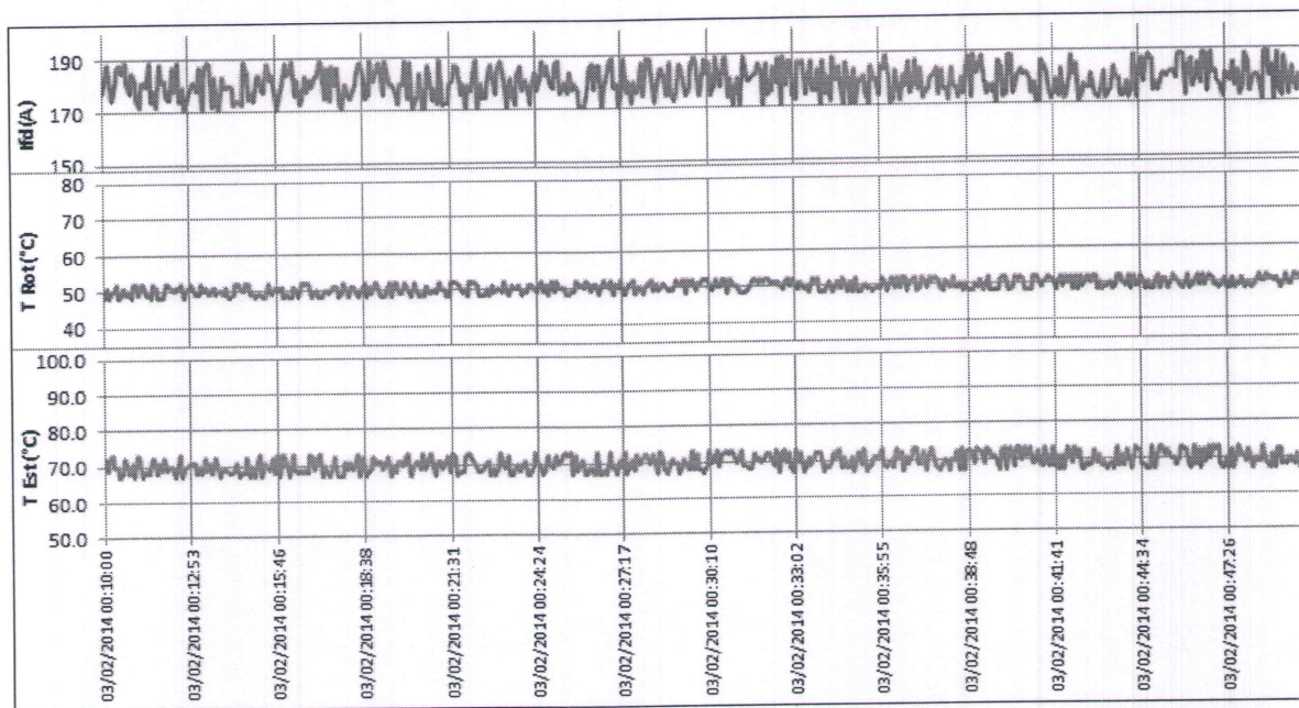
Figura 6-15: Registro Región Subexcitación – Mínimo Técnico
