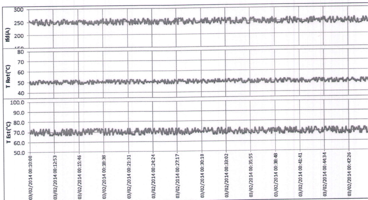
Figura 6-11: Registro Región Subexcitación – Potencia Nominal
