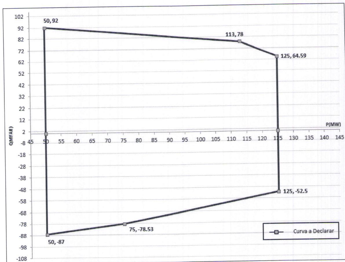
Figura 6-16 Curva de capacidad verificada
