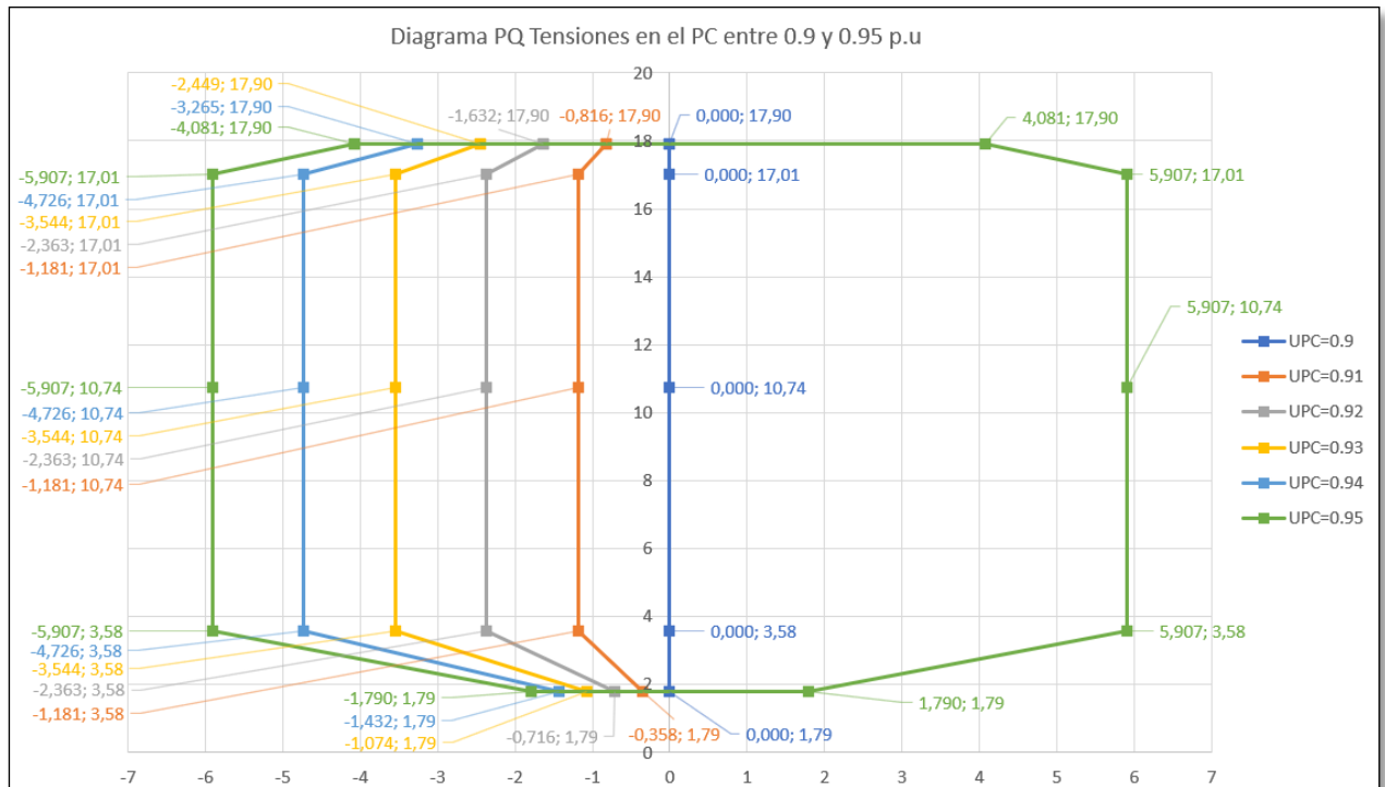
Figura 8.3 – Curva de capacidad con corrección por tensión. Zona de absorción.
