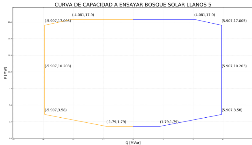
Figura 2.1 – Curva de capacidad a auditar.
