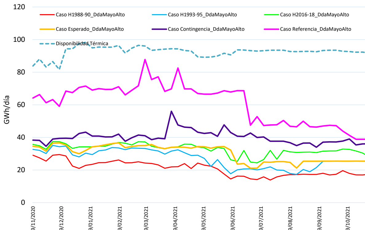
Gráfica 2 Generación térmica.
