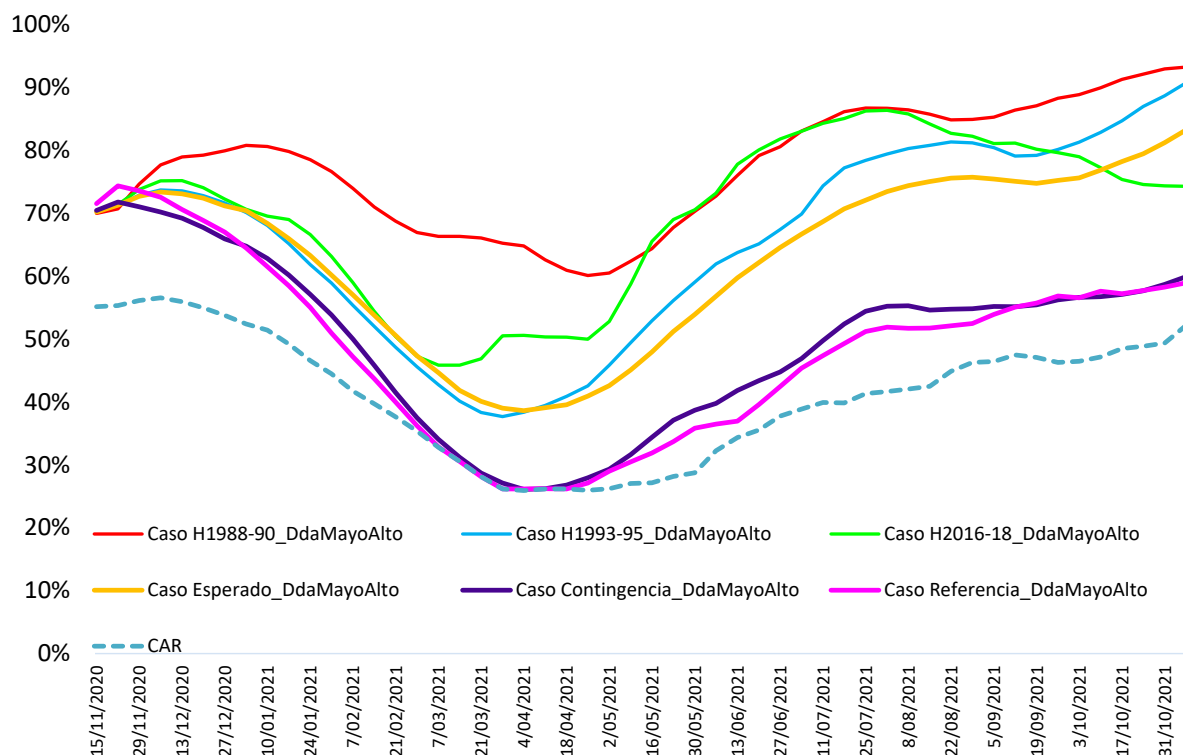
Gráfica 3 Volumen útil agregado del SIN.
