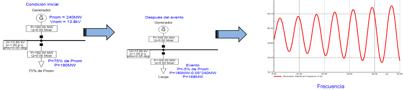
Figura A2.2 Ejemplo de sistema de prueba y definición del evento para simulación de respuesta en red aislada
