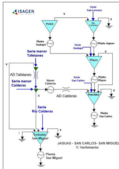
Topología centrales San Carlos y San Miguel
