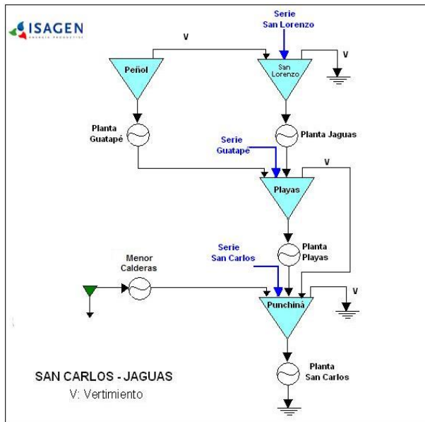
Topología anterior de la central San Carlos (embalse Punchiná)
