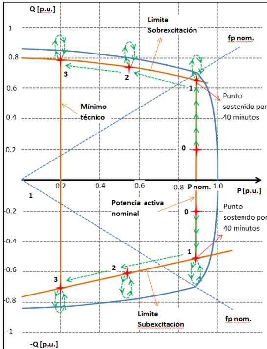
Figura 11. Esquema para la realización de las pruebas potencia reactiva de generadores
