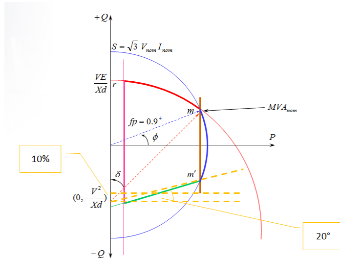
Figura 5. Margen de seguridad angular + margen de seguridad de tensión utilizados para determinar el límite práctico de estabilidad en generadores de polos lisos de acuerdo con la metodología 2 [3].
