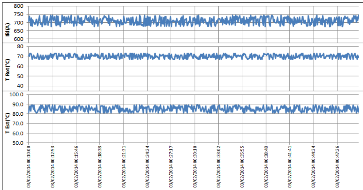
Figura 6-9: Registro Región Sobrexcitación – Mínimo Técnico
