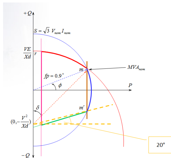
Figura 4. Margen de seguridad angular utilizado para determinar el límite práctico de estabilidad en generadores de polos lisos de acuerdo con la metodología 2 [3].
