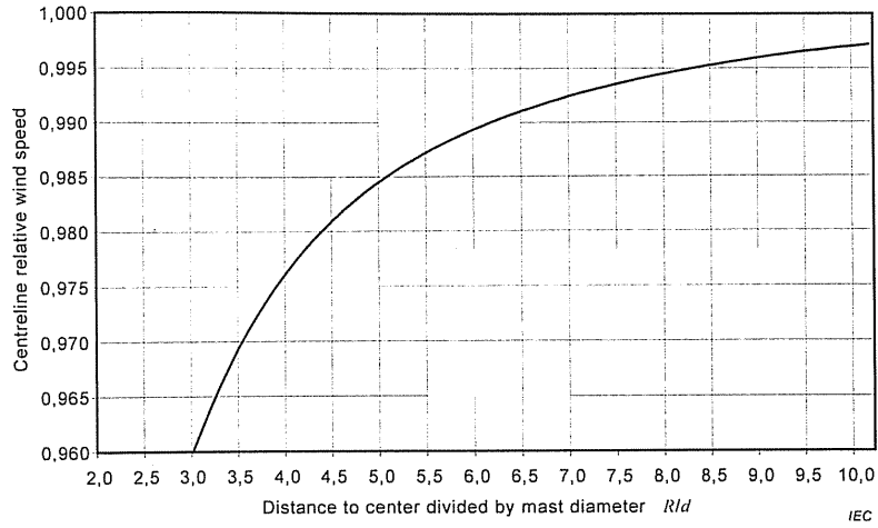
Figura 6: Velocidad relativa del viento en la línea central en función de la distancia R_d desde el centro de un mástil meteorológico tubular y el diámetro del mástil meteorológico d . Tomado de [1].
