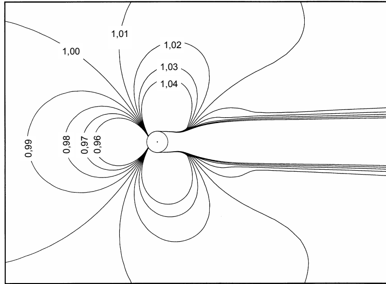
Figura 5: Isolneas de velocidad de flujo local alrededor de un mástil meteorológico tubular cilíndrico. Normalizado por la velocidad de flujo de campo libre. Tomado de [1].
