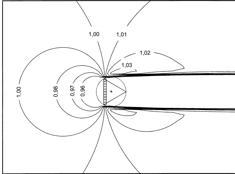
Figura 8: Isolíneas de velocidad de flujo local alrededor de un mástil meteorológico reticulado triangular con C_T de 0.5. Normalizado por la velocidad de flujo de campo libre. Tomado de [1].
