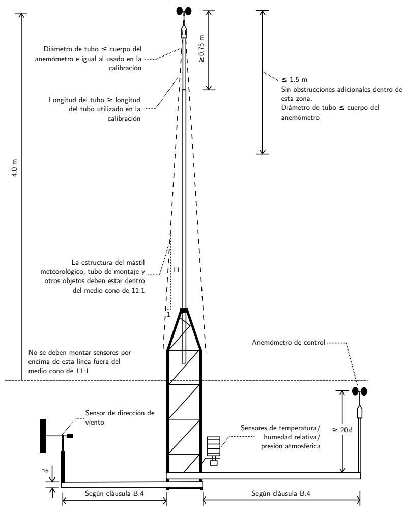
Figura 3: Ejemplo de anemómetro ubicado en la parte superior del mástil meteorológico y requerimientos de montaje. Adaptado de [1].
