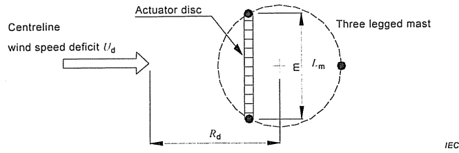
Figura 7: Representación de un mástil meteorológico reticulado de tres patas. Tomado de [1].
