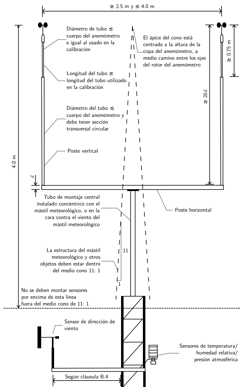
Figura 4: Ejemplo de anemómetros ubicados lado a lado en la parte superior del mástil meteorológico y requerimientos de montaje. Adaptado de [1].
