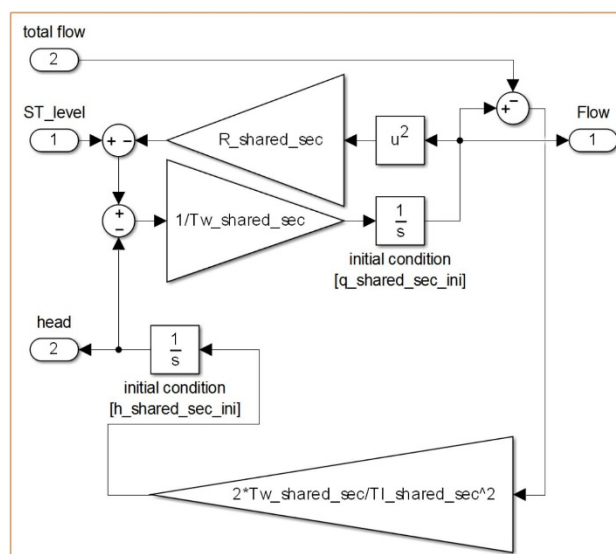
Figura 17. Modelo SIMULINK, bloque Penstock Shared
