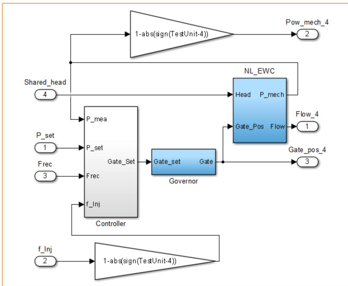
Figura 19. Modelo SIMULINK, bloque Unit 4 Regulator
