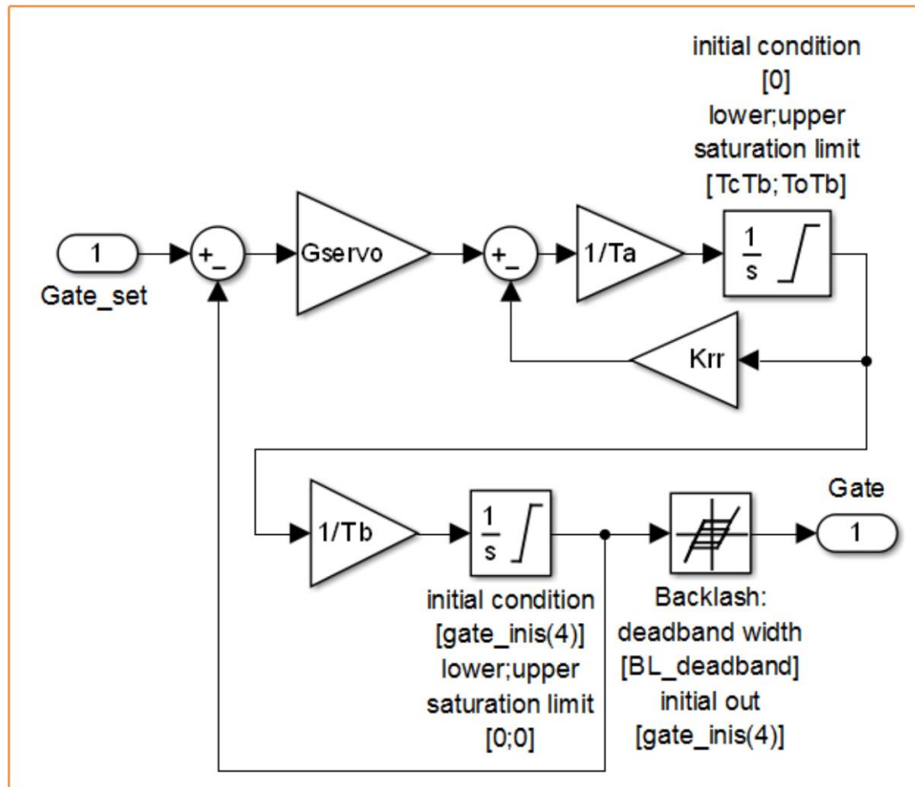
Figura 21. Modelo SIMULINK, bloque Unit 4 Regulator/Governor
