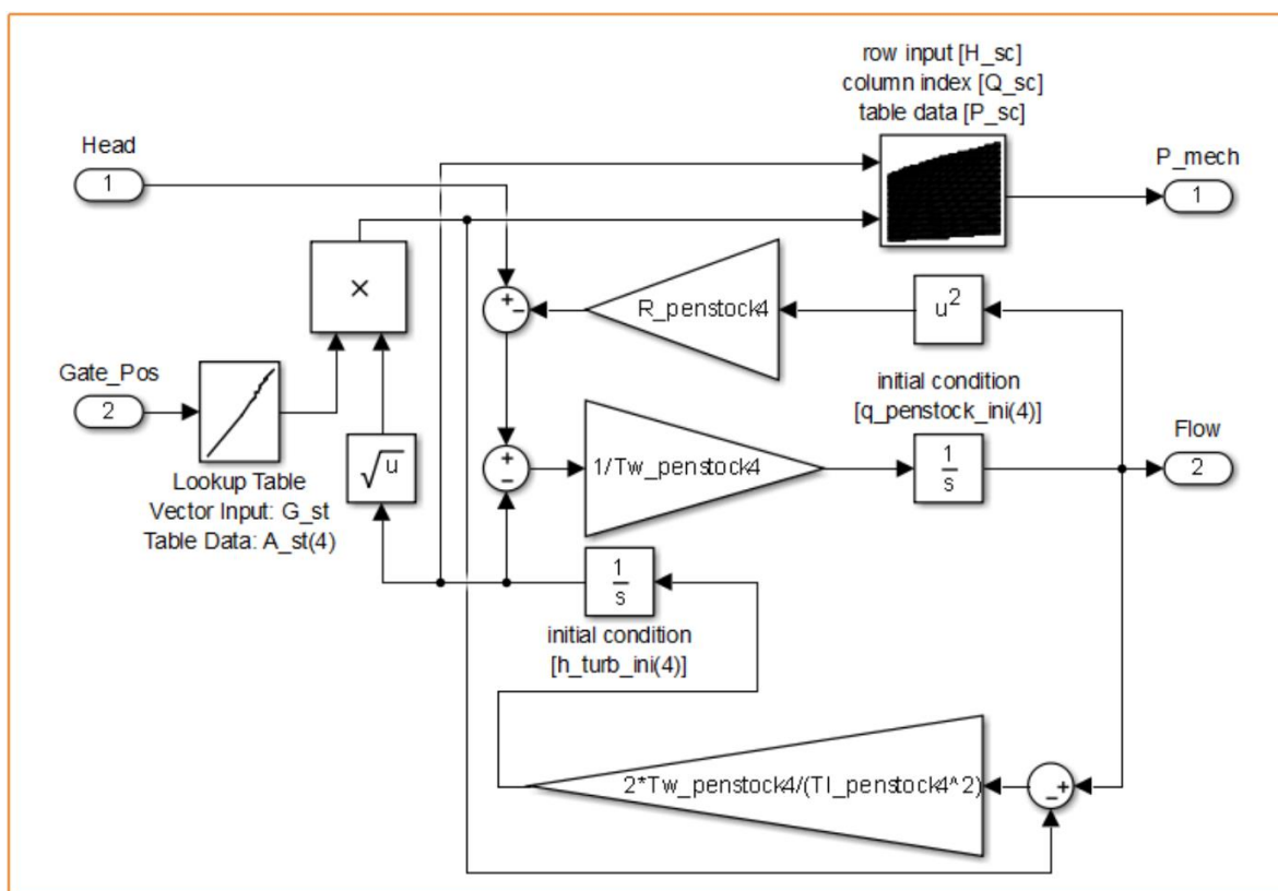
Figura 22. Modelo SIMULINK, bloque Unit 4 regulator/NL_EWC
