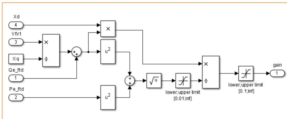
Figura 11. Modelo SIMULINK, bloque Automatic gain correction
