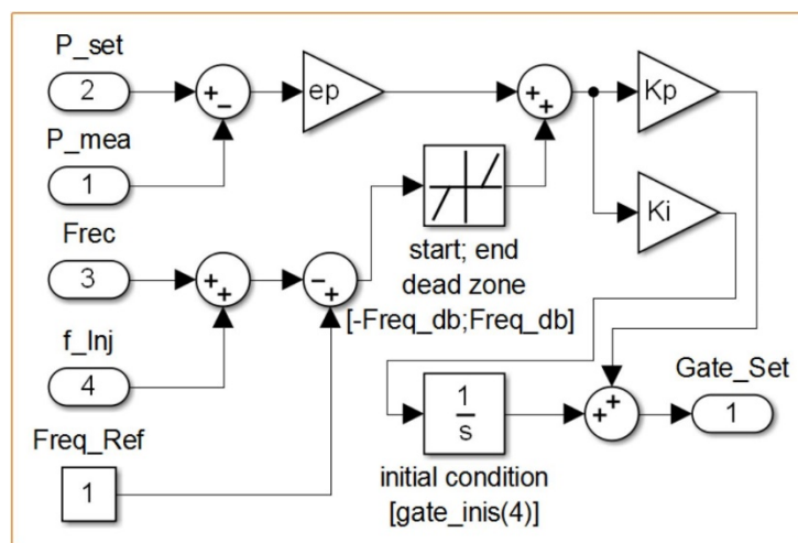
Figura 20. Modelo SIMULINK, bloque Unit 4 Regulator/Controller
