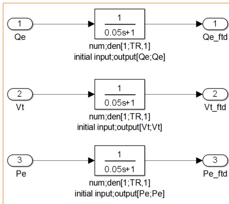
Figura 8. Modelo SIMULINK, bloque PQ_limiter
