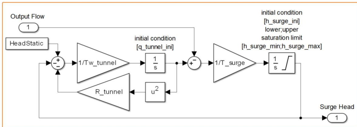
Figura 18. Modelo SIMULINK, bloque Surge Tank
