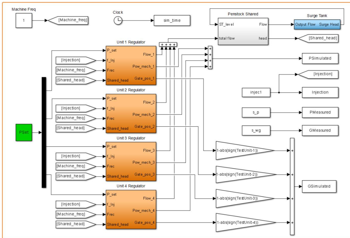
Figura 16. Modelo SIMULINK conjunto regulador de velocidad
