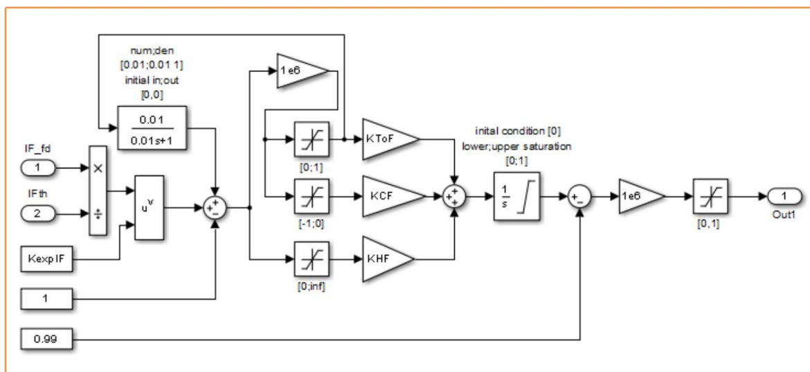
Figura 12. Modelo SIMULINK, bloque IFmax_limiter
