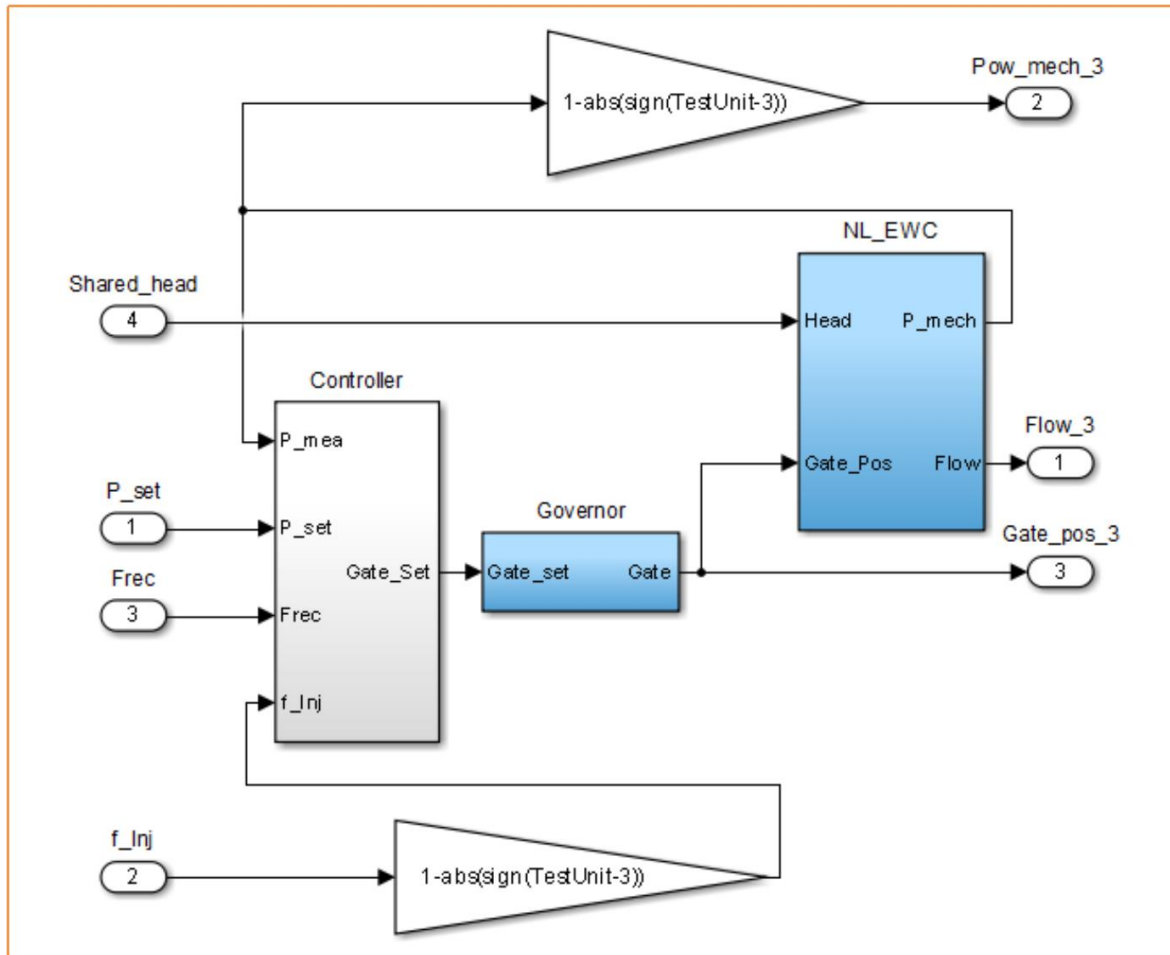
Figura 19. Modelo SIMULINK, bloque Unit 3 Regulator
