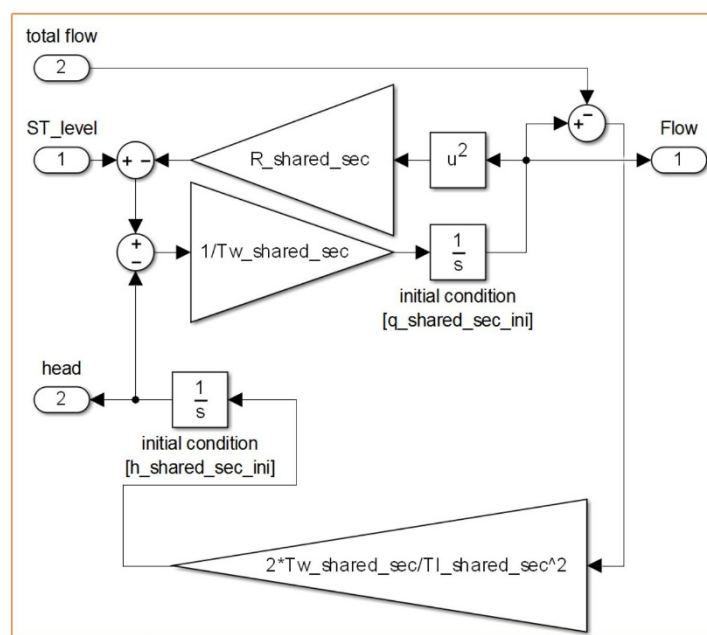
Figura 17. Modelo SIMULINK, bloque Penstock Shared
