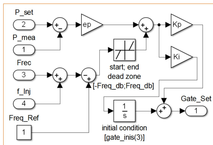
Figura 20. Modelo SIMULINK, bloque Unit 3 Regulator/Controller
