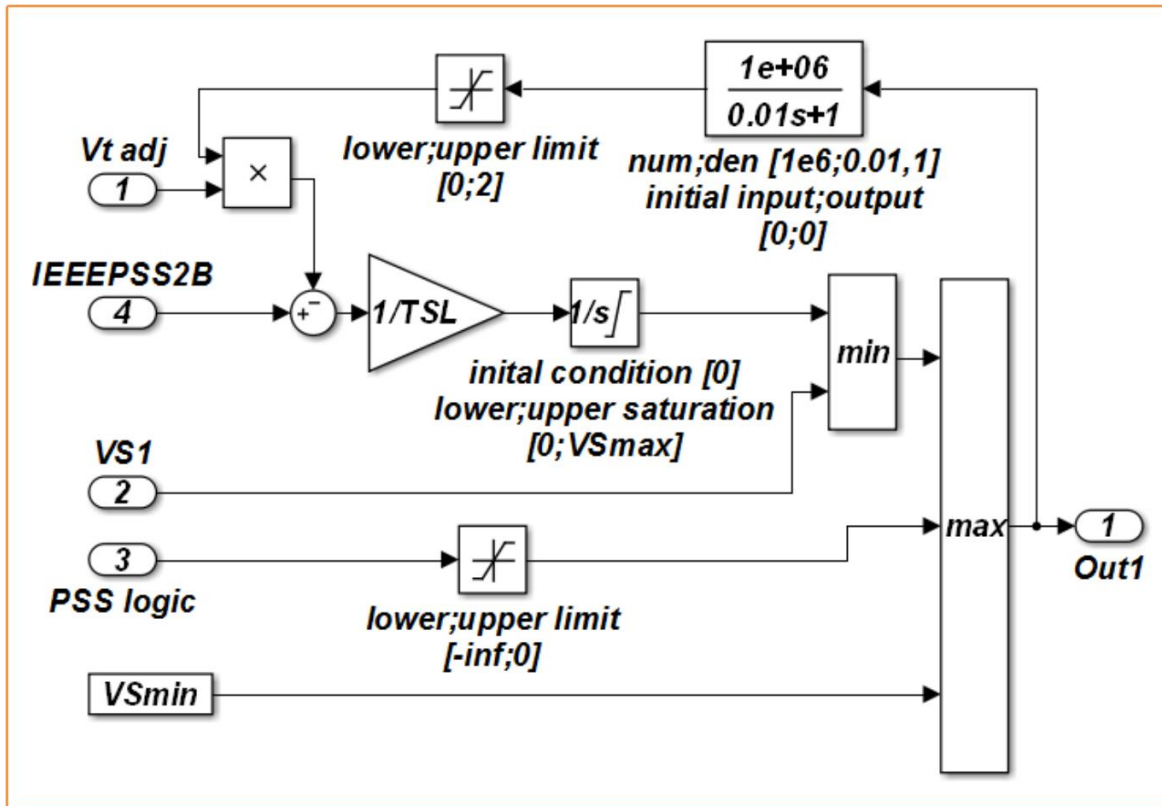
Figura 7. Modelo SIMULINK, bloque ramp_adjust
