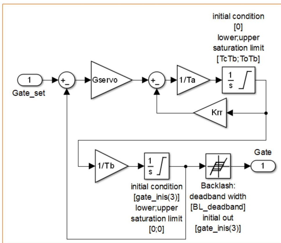
Figura 21. Modelo SIMULINK, bloque Unit 3 Regulator/Governor
