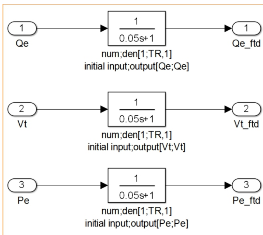
Figura 9. Modelo SIMULINK, bloque Filter measurement
