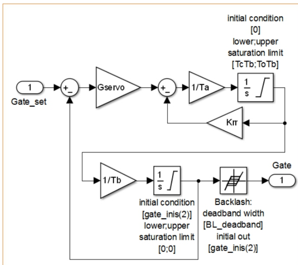
Figura 21. Modelo SIMULINK, bloque Unit 1 Regulator/Governor
