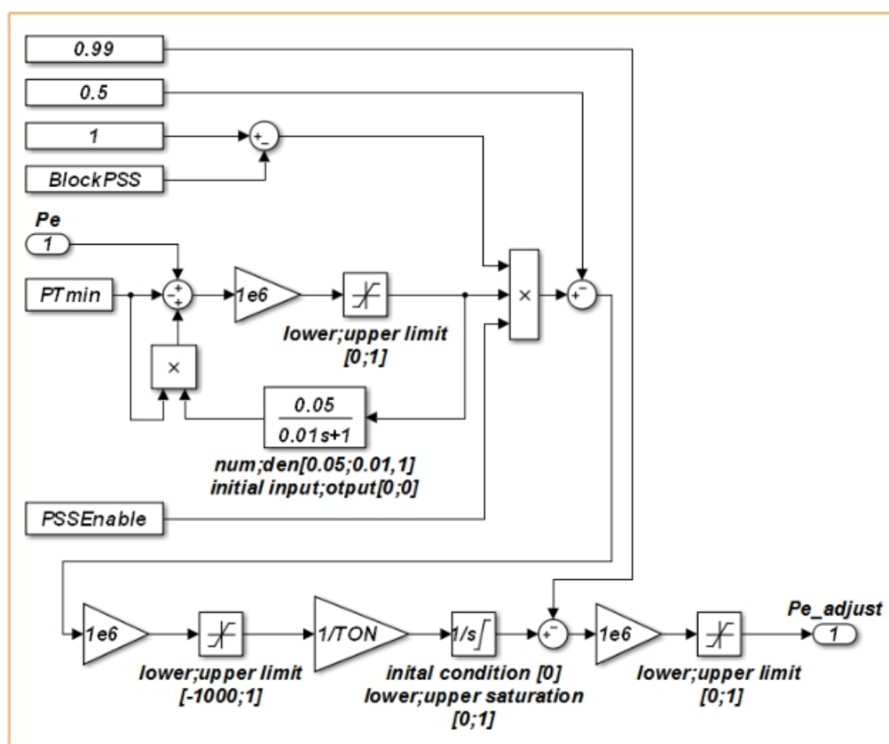
Figura 4. Modelo SIMULINK, bloque Pe adjust.
