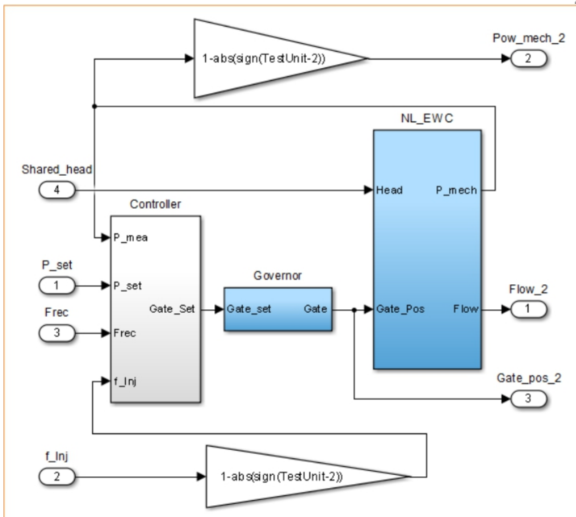
Figura 19. Modelo SIMULINK, bloque Unit 2 Regulator
