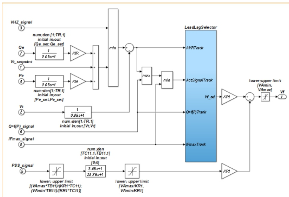
Figura 2. Modelo SIMULINK, bloque AVR
