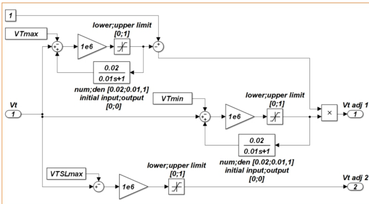
Figura 6. Modelo SIMULINK, bloque VT adjust
