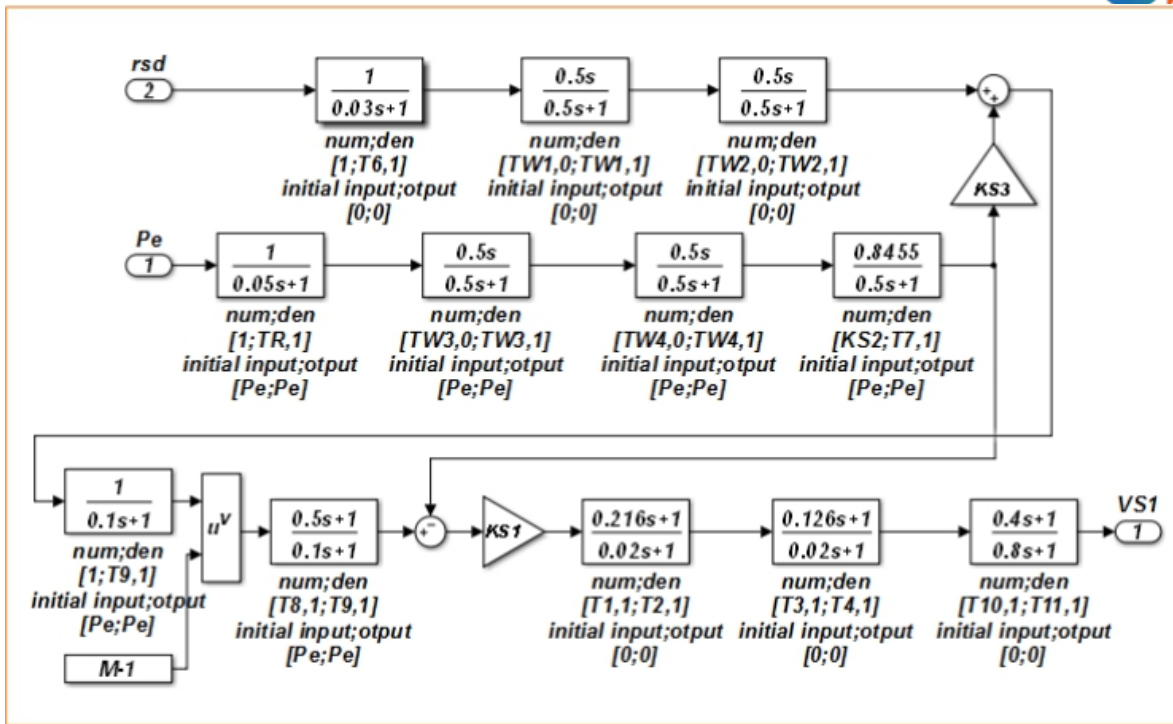
Figura 5. Modelo SIMULINK, bloque PPS 2B
