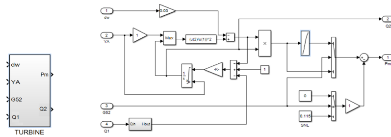
Figura 3: Bloque de control turbina y conducción
