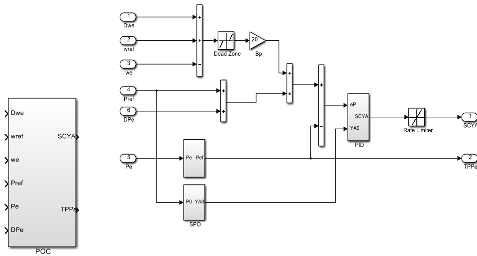
Figura 1: Bloque de control módulo POC
