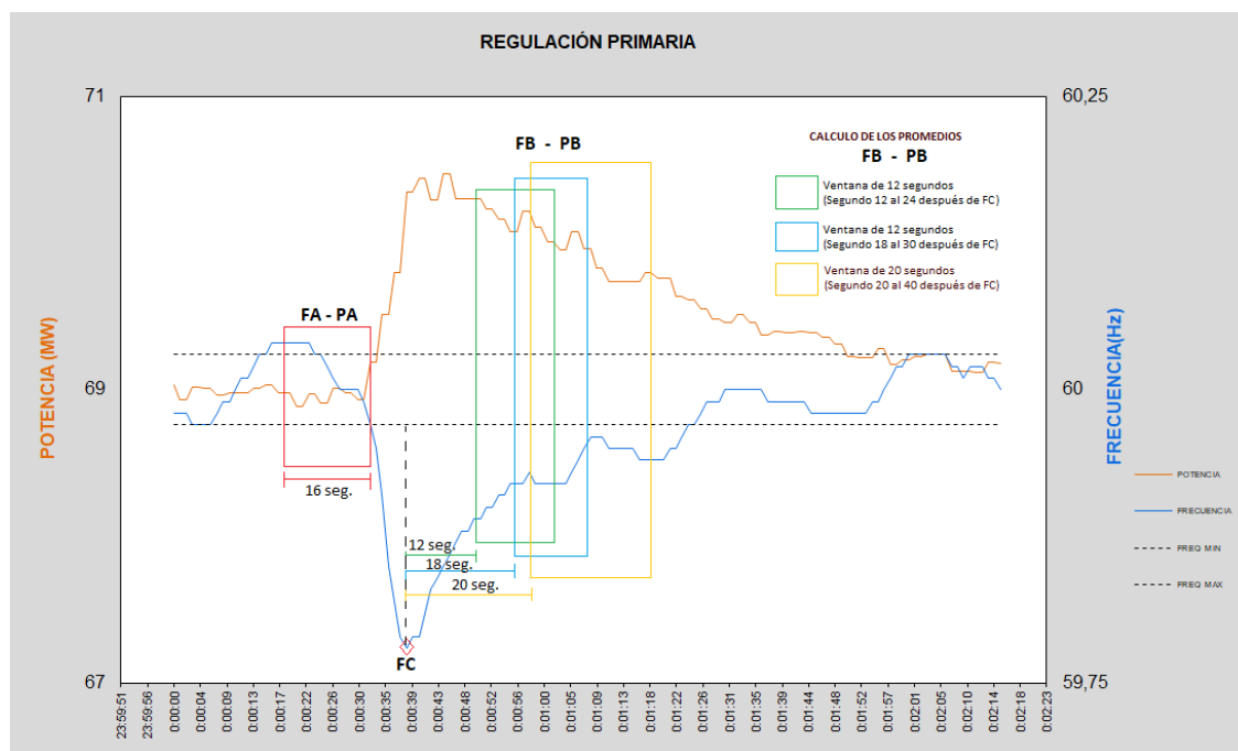
Figura 6. Períodos para estimar el estatismo.
