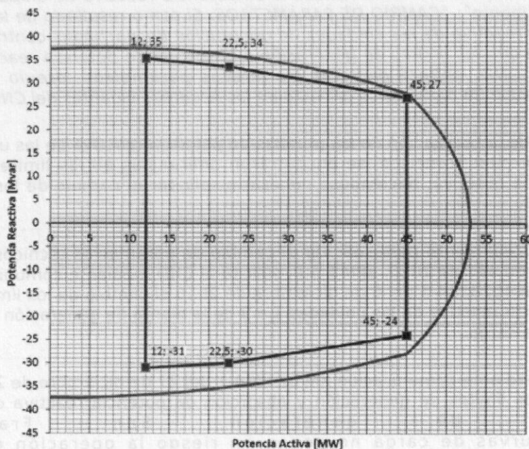
Curva de cargabilidad unidades 1 a 3 San Francisco
