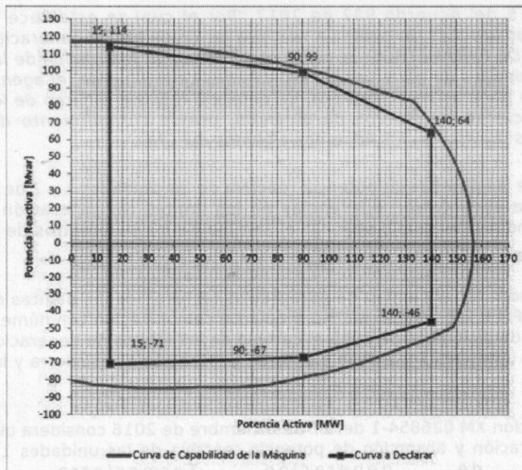
Curva de cargabilidad unidades 1 y 2 Termosierra
