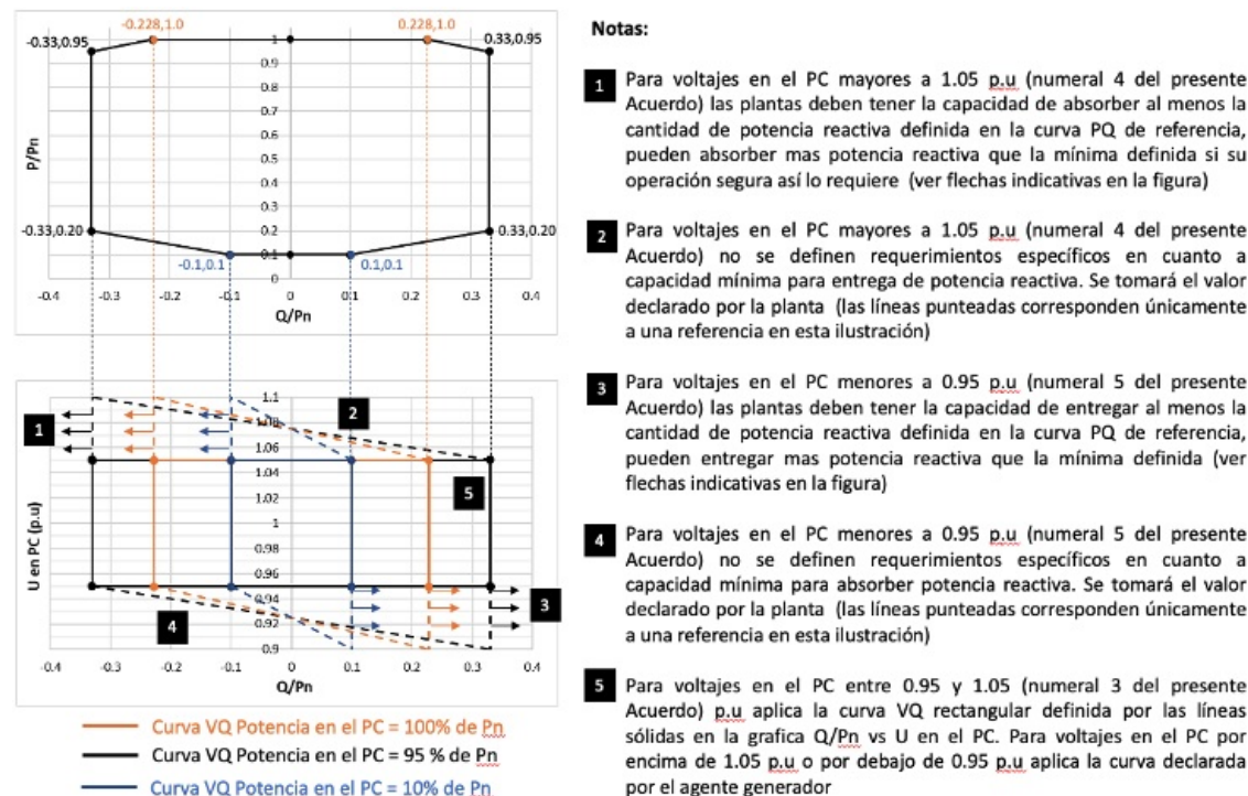
Figura 2: Curva PQ de referencia definida en la Resolución CREG 148 de 2021 y su relación con la curva VQ definida para las plantas objeto de este Acuerdo
