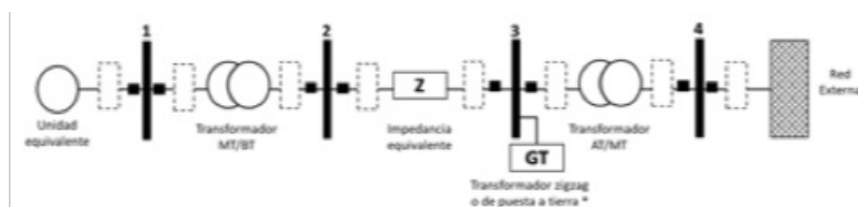
Figura 1. Diagrama unifilar para modelo eléctrico de generadores eólicos y solares conectados al STN, STR y SDL
