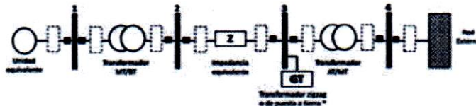
Figura 1. Diagrama unifilar para modelo eléctrico de generadores eólicos y solares conectados al STN, STR y SDL
