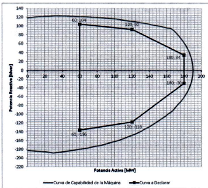
Figura 1. Curva de Carga Unidad 2 de la central Betania
