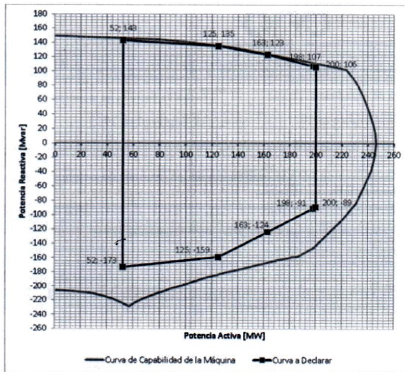
Figura 1. Curva de Carga Unidades 1 y 2 de la central Químbo
