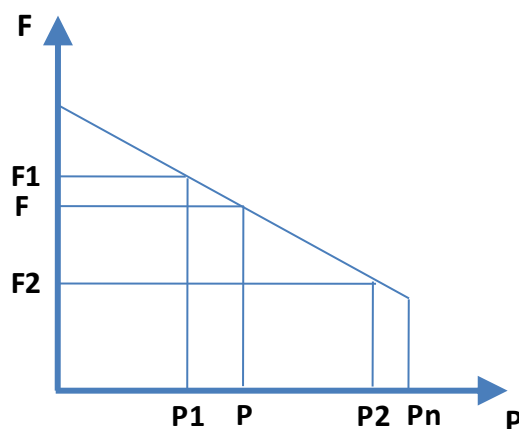
Figura 2. Estadismo de una Unidad de Generación
