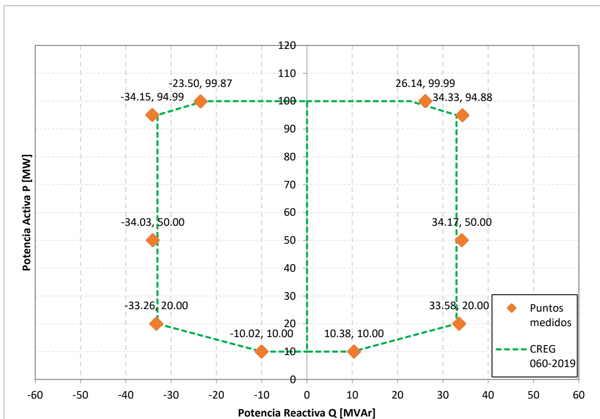
Gráfico 4. Curva de capacidad a declarar de la PSFV La Unión
