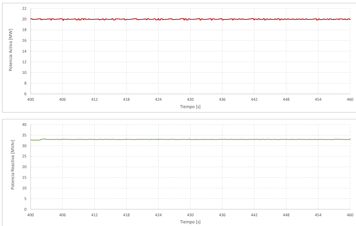
Gráfico 15. Registro de potencia activa y potencia reactiva. PQ 2. Control Q
