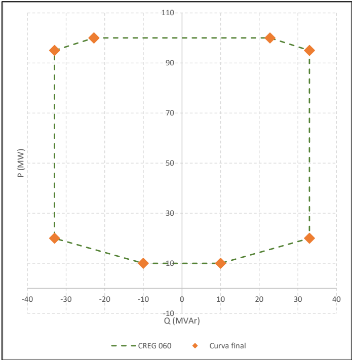
Gráfico 37. Curva PQ a declarar por parte de la planta.
