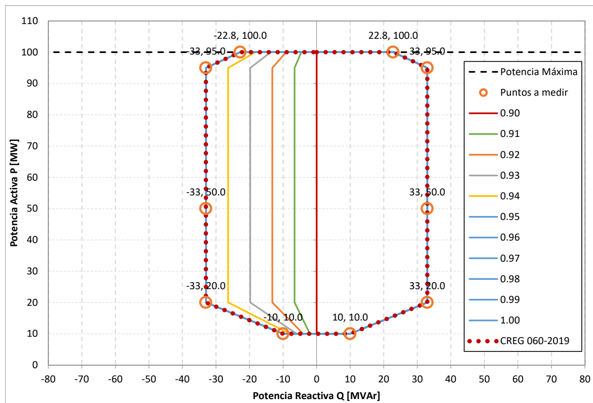
Gráfico 2. Curva de capacidad (PQ) propuesta en el POI entre 0,90 y 1,00 pu
