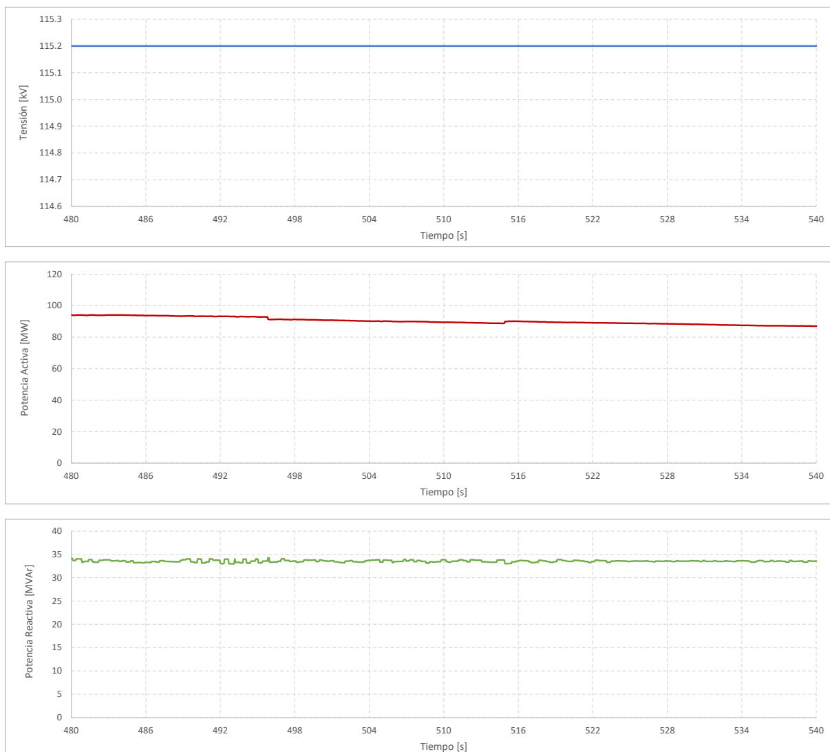
Gráfico 27. Registro de potencia activa y potencia reactiva. PQ 4. Control Q
