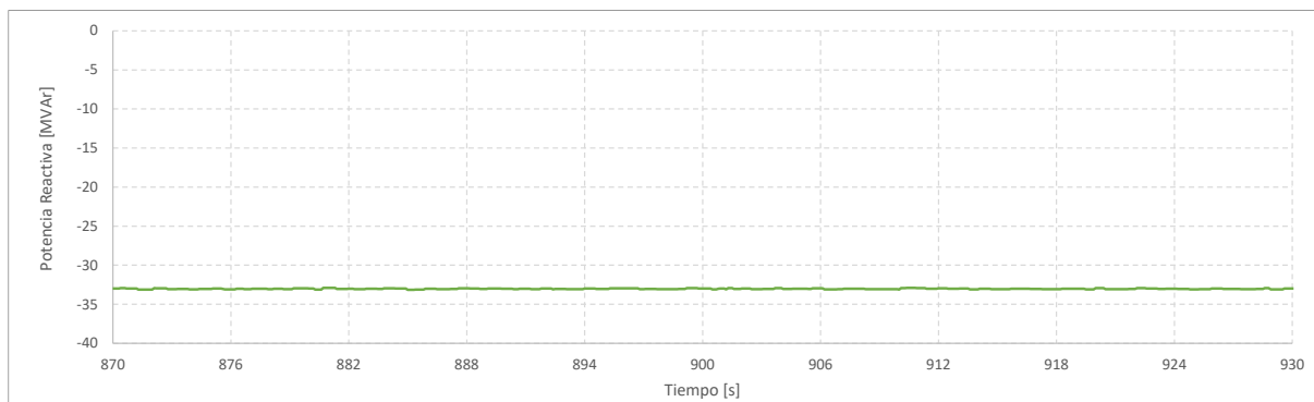
Gráfico 17. Registro de potencia activa y potencia reactiva. PQ 9. Control FP
