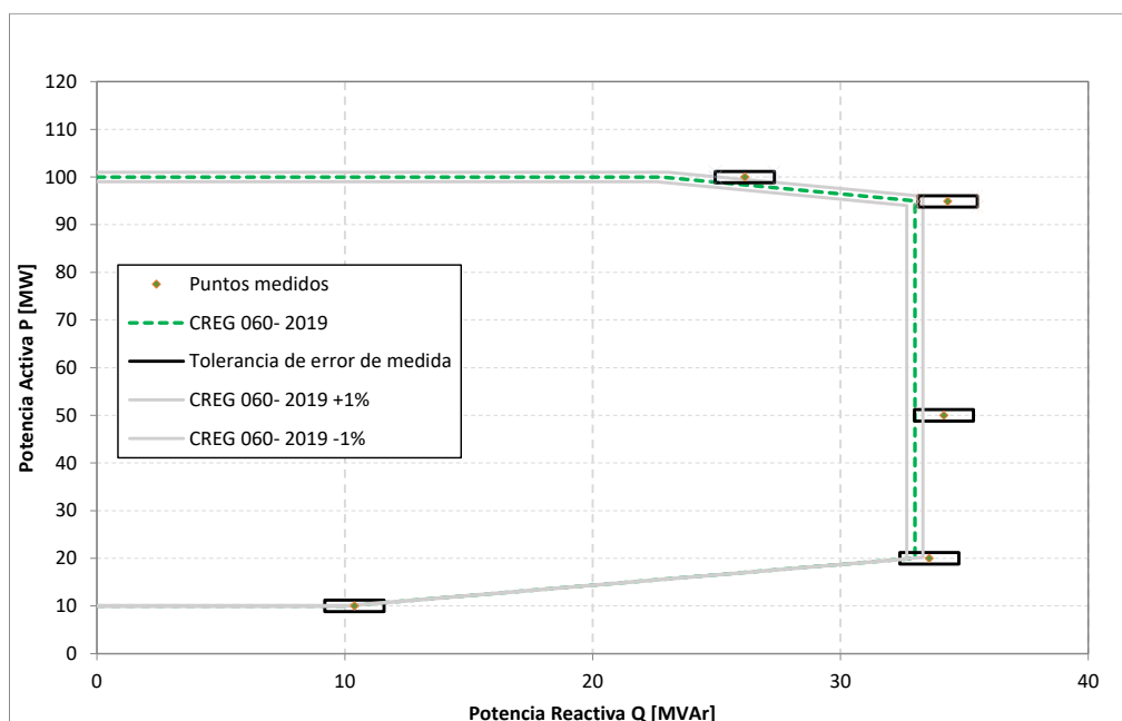
Gráfico 5. Detalle de región de entrega de potencia reactiva
