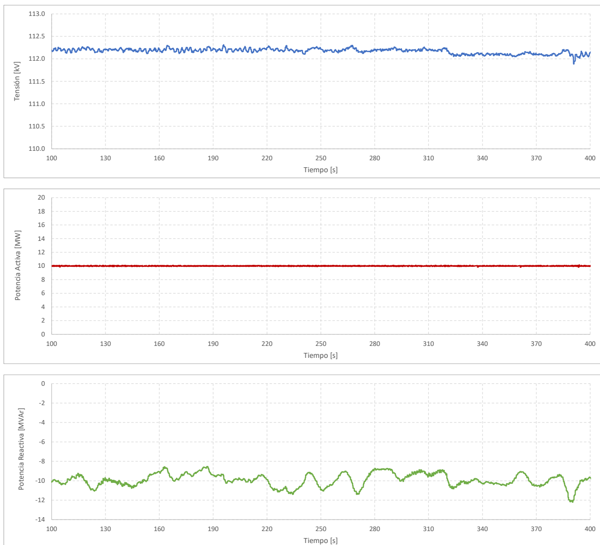
Gráfico 10. Registro de potencia activa y potencia reactiva. PQ 10. Control V
