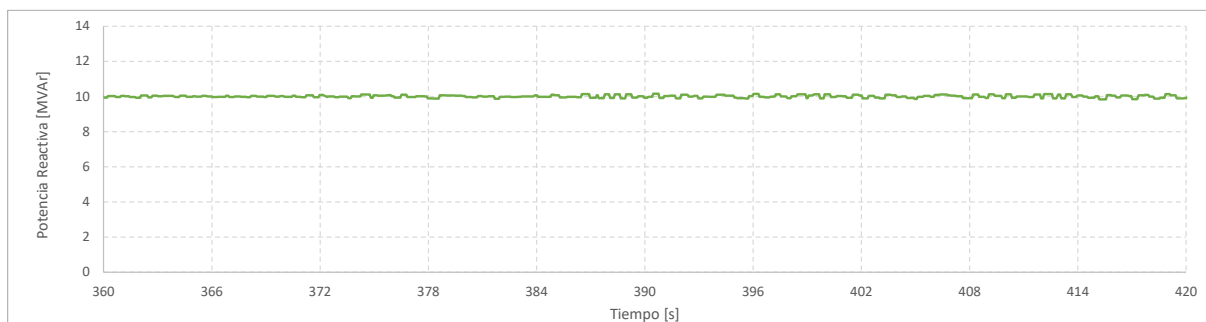
Gráfico 9. Registro de potencia activa y potencia reactiva. PQ 1. Control Q
