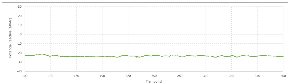
Gráfico 34. Registro de potencia activa y potencia reactiva. PQ 6. Control V
