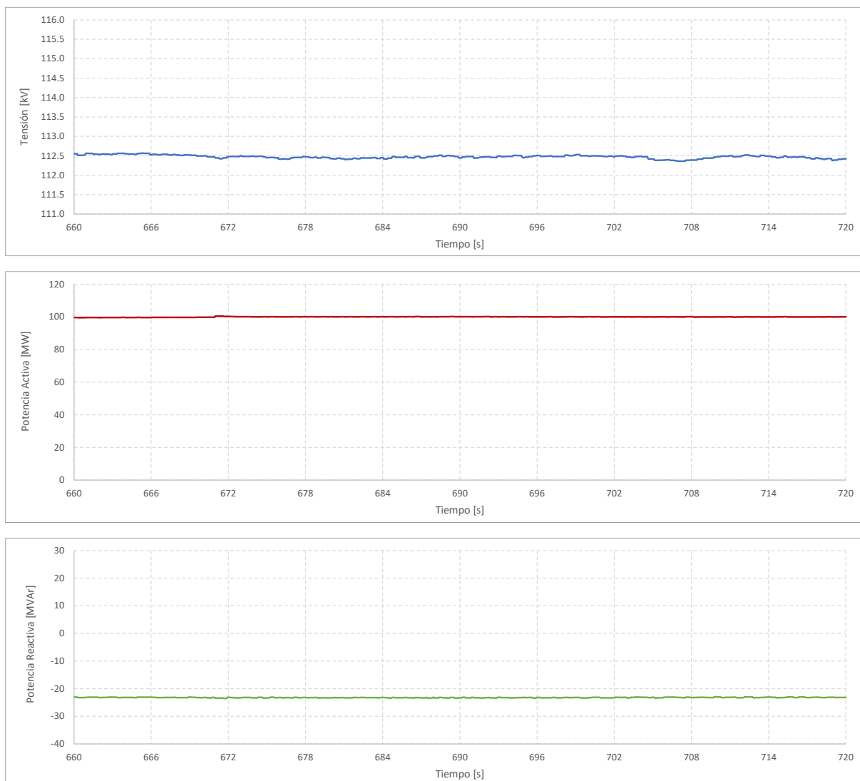
Gráfico 35. Registro de potencia activa y potencia reactiva. PQ 6. Control FP
