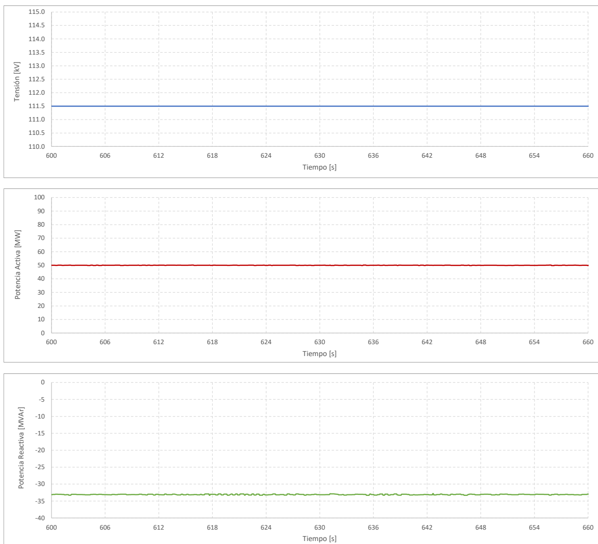
Gráfico 23. Registro de potencia activa y potencia reactiva. PQ 8. Control FP
