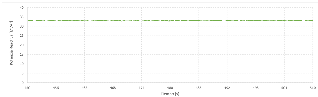
Gráfico 21. Registro de potencia activa y potencia reactiva. PQ 3. Control Q
