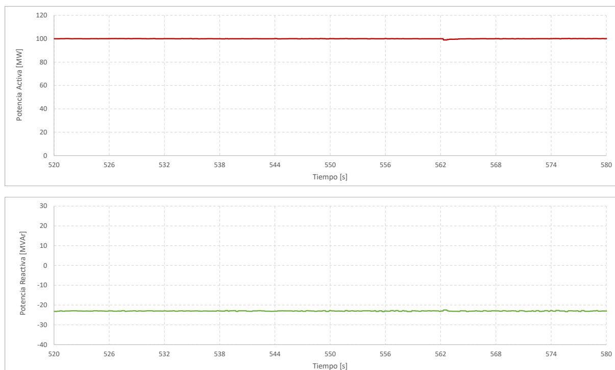
Gráfico 36. Registro de potencia activa y potencia reactiva. PQ 6. Control Q
