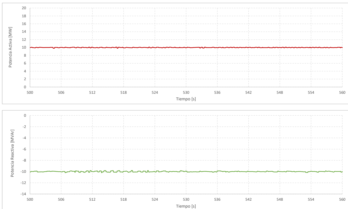
Gráfico 11. Registro de potencia activa y potencia reactiva. PQ 10. Control FP
