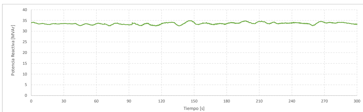
Gráfico 13. Registro de potencia activa y potencia reactiva. PQ 2. Control V
