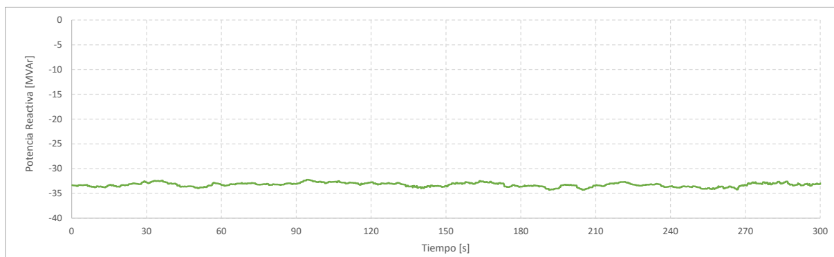
Gráfico 16. Registro de potencia activa y potencia reactiva. PQ 9. Control VQ
