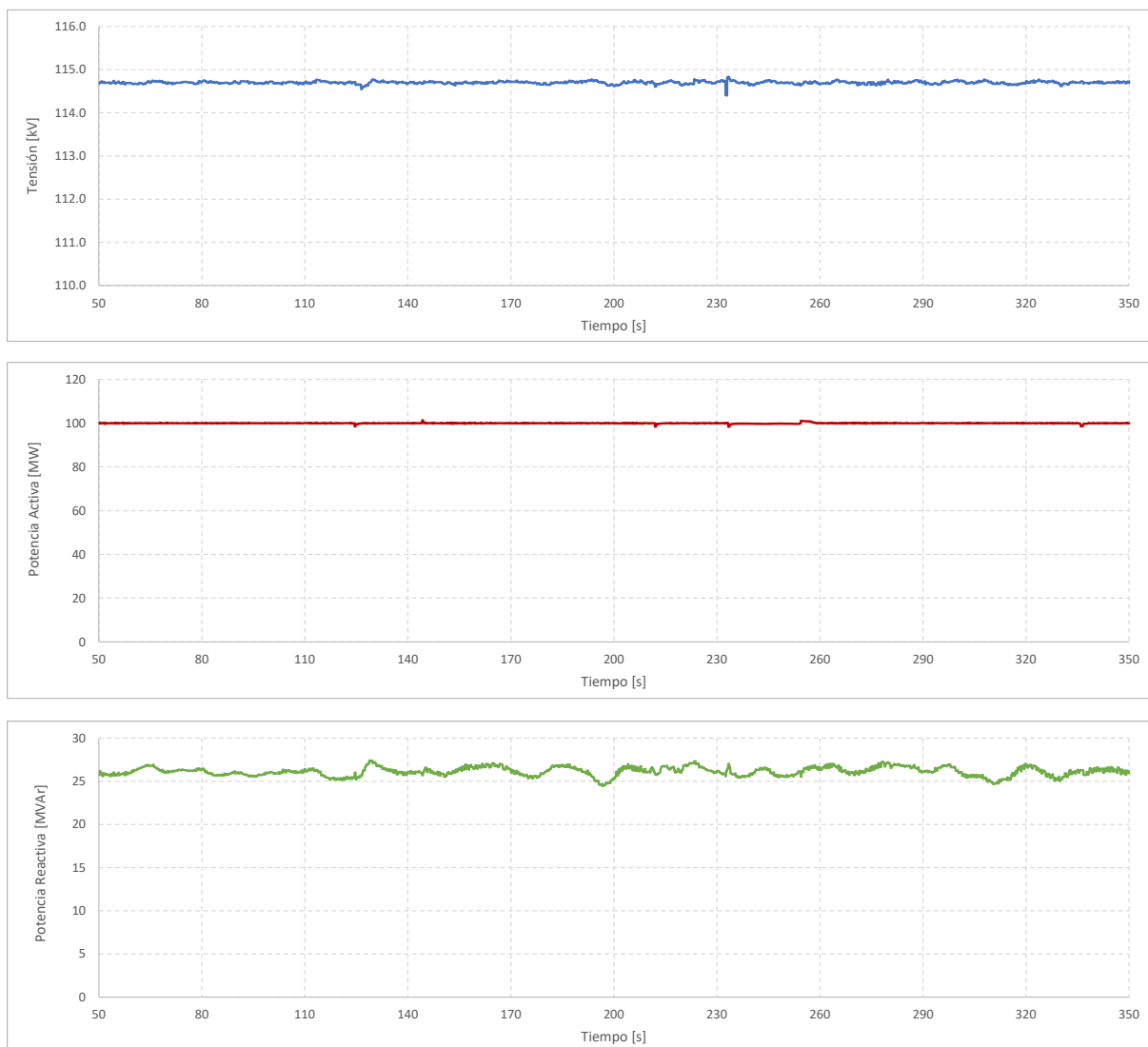
Gráfico 31. Registro de potencia activa y potencia reactiva. PQ 5. Control V
