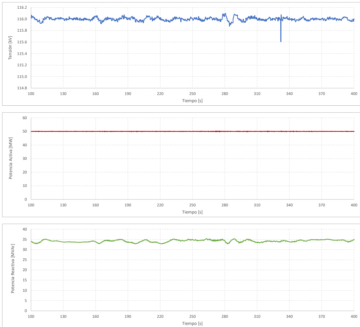
Gráfico 19. Registro de potencia activa y potencia reactiva. PQ 3. Control V
