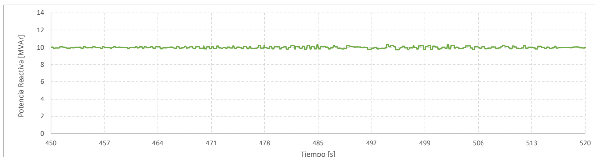
Gráfico 8. Registro de potencia activa y potencia reactiva. PQ 1. Control FP
