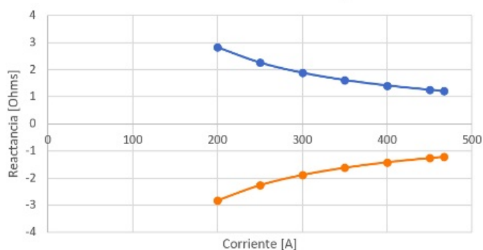
Valores Posibles de Reactancia Inyectada
