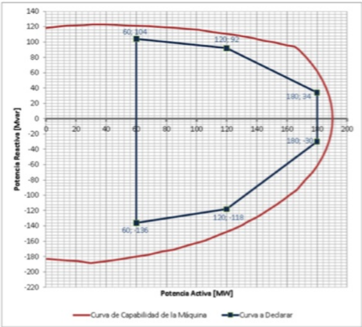
Figura 1. Curva de Carga Unidad 1 de la central Betania
