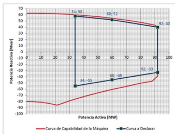
Figura 3. Curva de Carga Unidades de la central Paraíso
