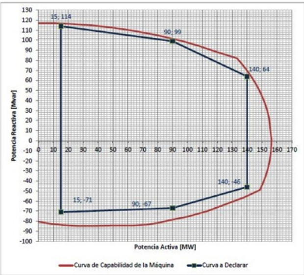
Curva de cargabilidad unidades 1 y 2 Termosierra
