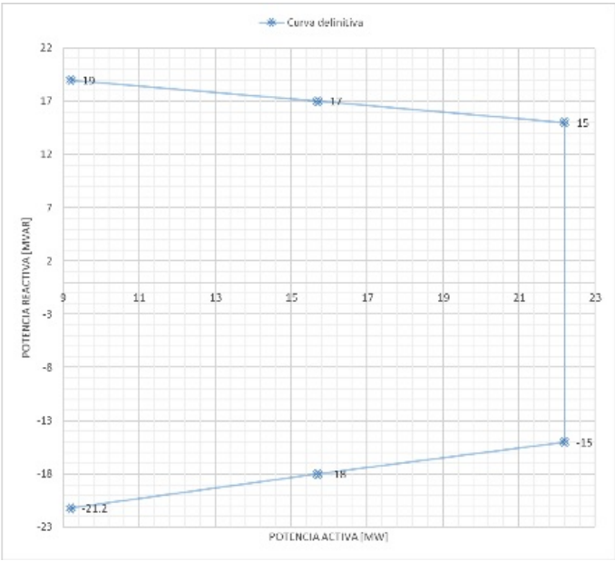
Curva de cargabilidad CH San Miguel
