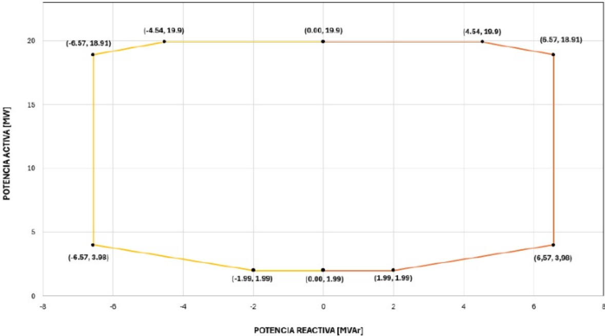
Curva de capacidad a ensayar - P.F. Planeta Rica
