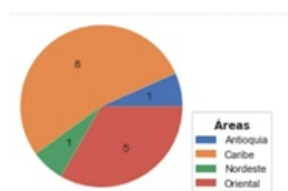
Figura 1. Subestaciones con capacidad de corto superior a la nominal – 1 enero 2024
