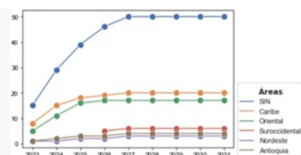
Figura 2. Subestaciones con capacidad de corto superior a la nominal – 2024 a 2031
