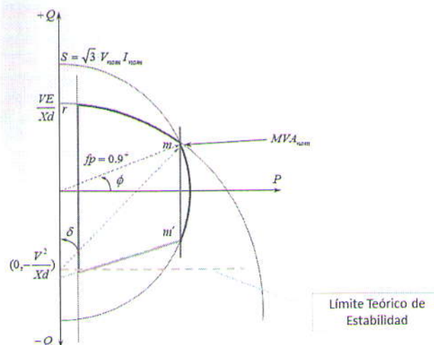
Figura 1. Cálculo del límite de estabilidad teórico para generadores de polos lisos de acuerdo con la metodología 2 [3].
