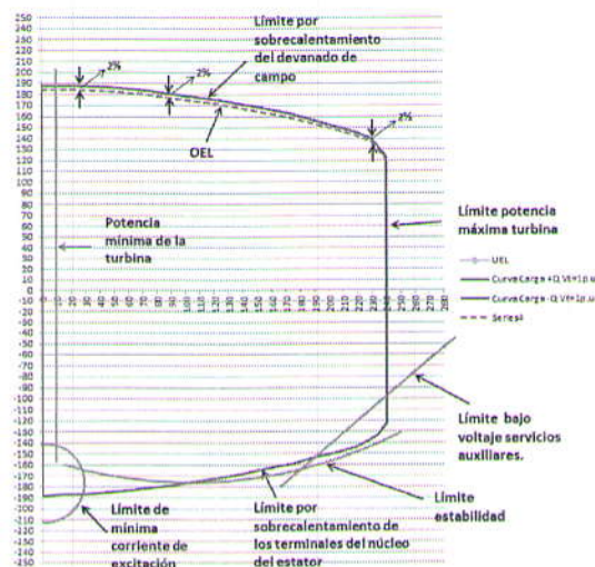
Figura 10. Ejemplo de Coordinación del limitador de sobrexcitación y la curva de carga
