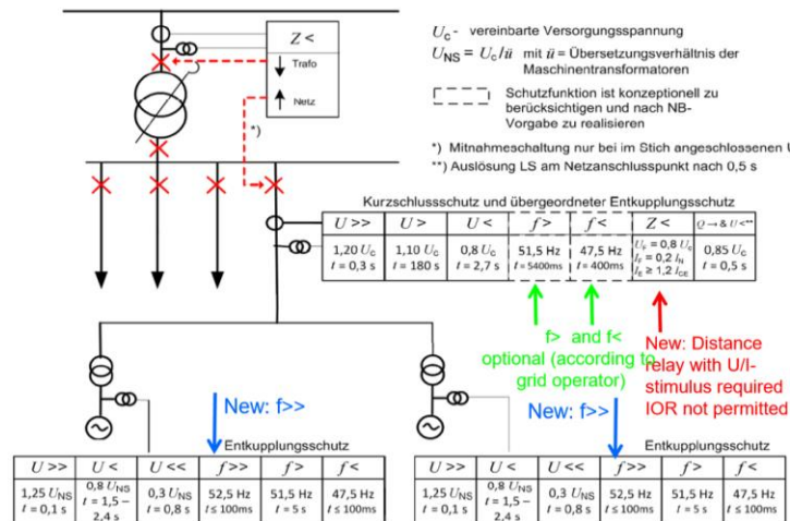
Figura 16. Funciones de protección recomendadas para GD conectada a media tensión [10].
