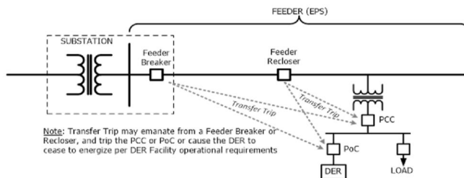
Figura 22. Ejemplo de esquema de disparo transferido a sistemas de generación [11].
