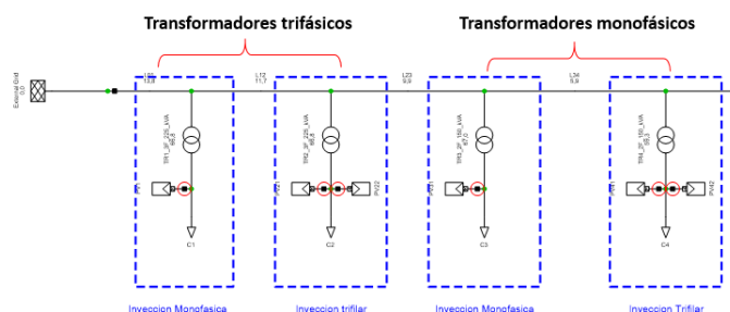
Figura 24. Conexiones monofásicas en transformadores
