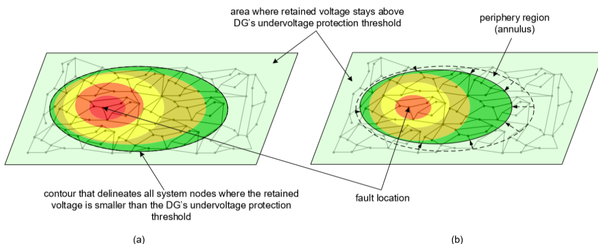
Figura 17. Ilustración del contorno de la tensión en redes del SDL (a) Modelo aproximado (b) Modelo simplificado [12]
