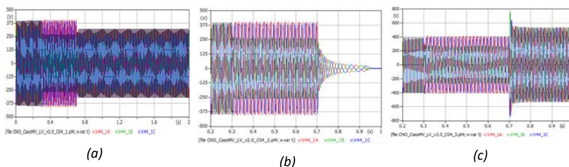
Figura 10. Caso 3 Tensión Fase-Tierra en Inversor (a) Carga 700 kW (b) Carga 1200 kW (c) Carga 300 kW
