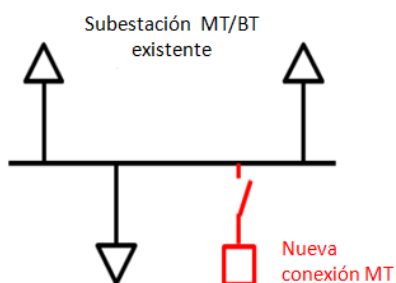
Figura 9 Derivación en T ramificada con seccionamiento.
