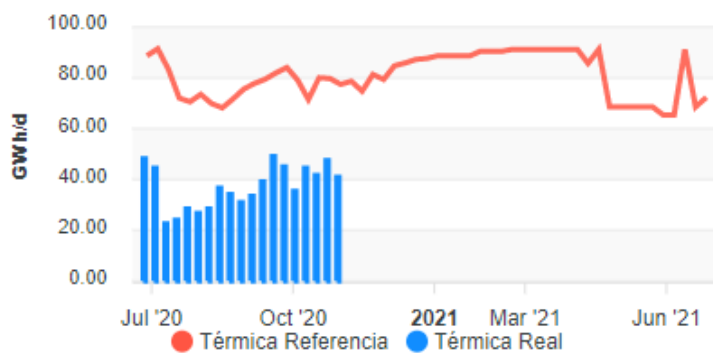
Gráfica 8 Evolución agregada generación térmica.
