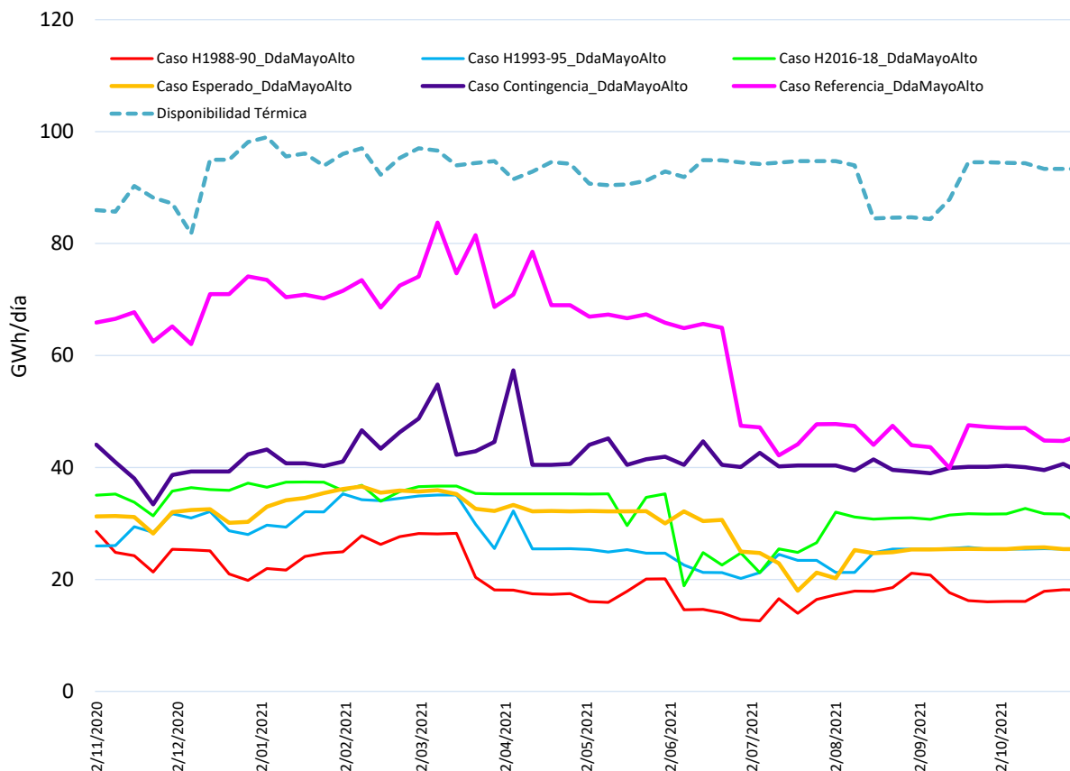
Gráfica 2 Generación térmica.
