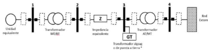
Figura 2. Diagrama unifilar para modelo eléctrico de generadores eólicos y solares conectados al STN, STR y SDL
