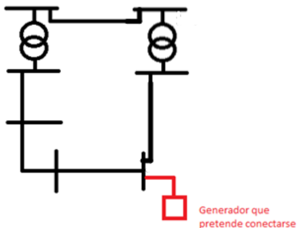
Figura 1 Red enmallada de referencia.
