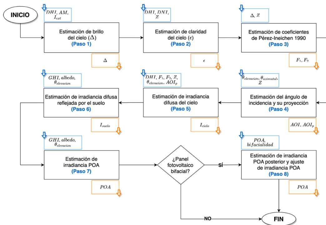
Figura 5.4. Diagrama de flujo del modelo de transposición Pérez-Ineichen 1990.
