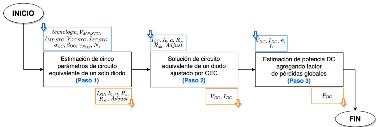
Figura 7.1. Diagrama de flujo de la producción DC.
