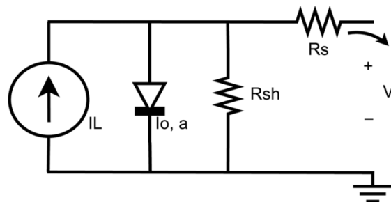
Figura 7.2. Circuito equivalente de un solo diodo par la estimación de la producción DC. Ilustración tomada de Dobos (2012) [6].
