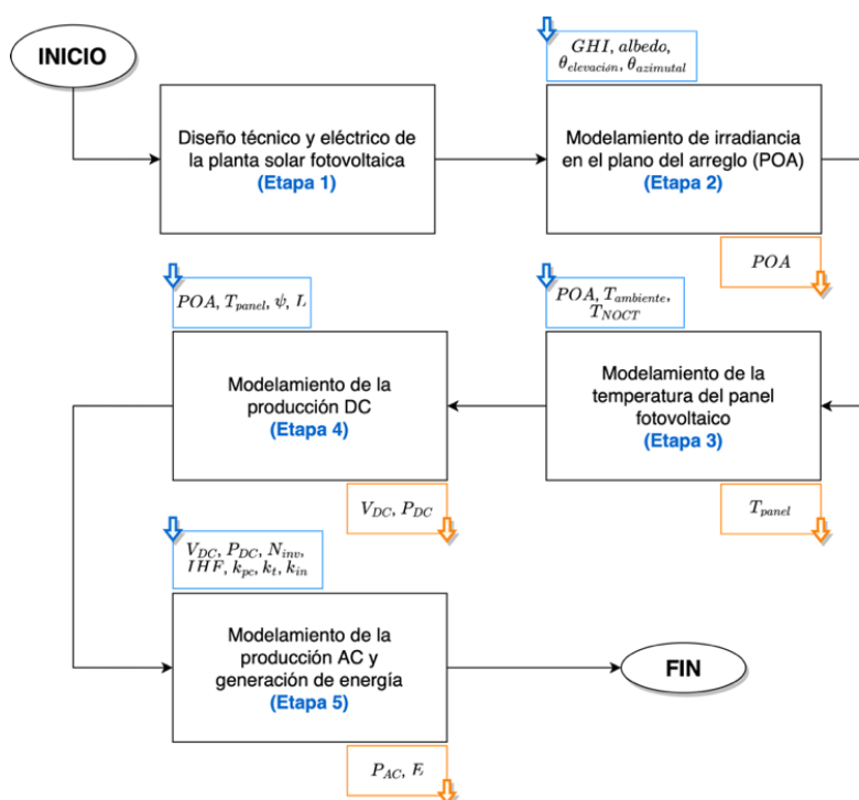
Figura 3.1. Diagrama de flujo general del modelo CNO de una planta solar fotovoltaica.
