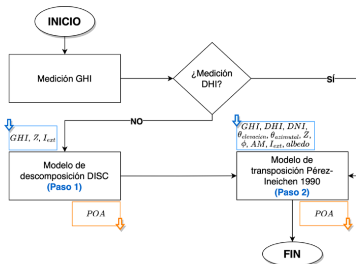
Figura 5.1. Diagrama de flujo para estimación de irradiancia en plano de arreglo (POA).
