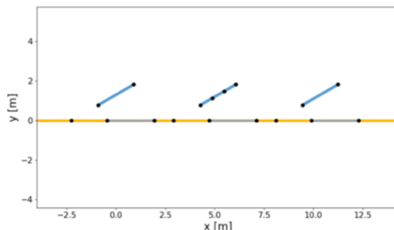
Figura 5.6. Tres filas de paneles fotovoltaicos (líneas azules) con seguidor de un eje orientados de norte a sur en un ángulo de rotación de 30°. Las líneas amarillas representan el suelo sin sombra, mientras que las líneas grises representan el suelo sombreado por los paneles fotovoltaicos. Ilustración tomada de [4].
