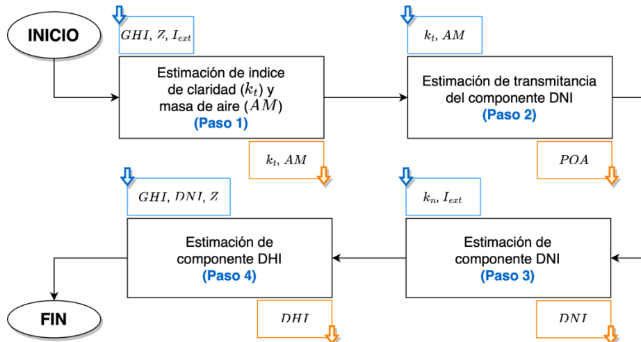
Figura 5.2. Diagrama de flujo del modelo de descomposición DISC.
