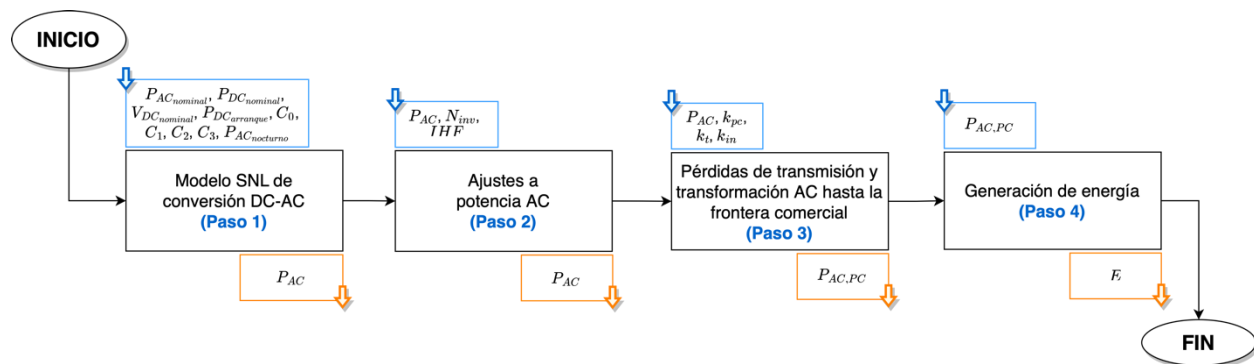
Figura 8.1. Diagrama de flujo de la producción AC y generación de energía.
