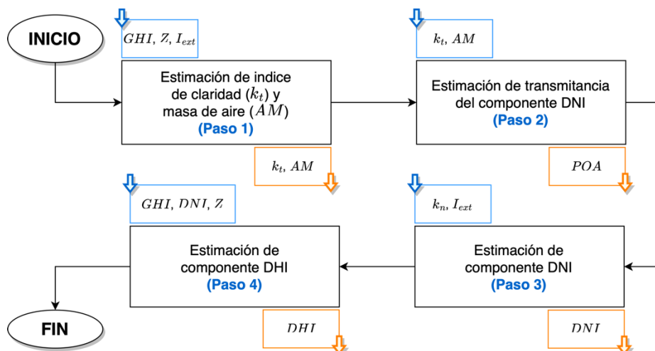
Figura 5.2. Diagrama de flujo del modelo de descomposición DISC.
