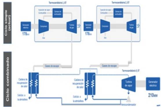
Proceso de generación térmica, Termocandelaria Ciclo Combinado
