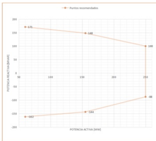
Figura 3: Curva de Carga Unidad 5 Central Guavio
