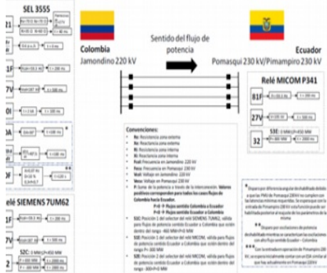
Figura 3-3. Ajustes de los Esquemas de Separación de Áreas vigentes en Colombia y Ecuador. Flujo Colombia - Ecuador
