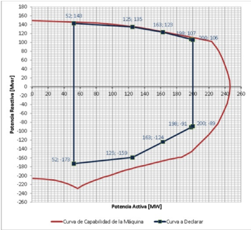
Figura 1. Curva de Carga Unidades 1 y 2 de la central Quimbo
