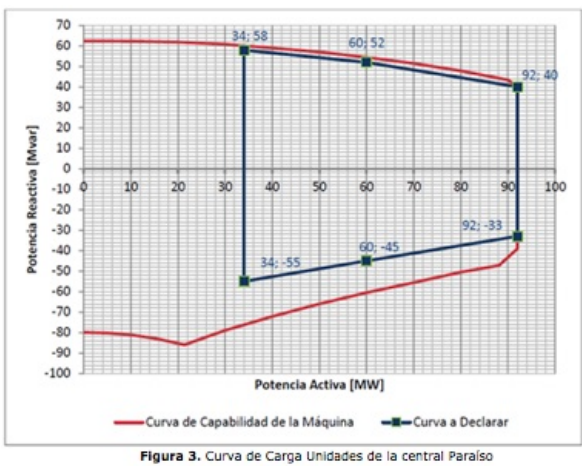
Figura 3. Curva de Carga Unidades de la central Paraíso
