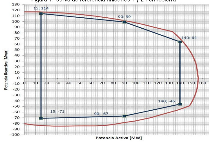
Figura 1. Curva de referencia unidades 1 y 2 Termosierra
